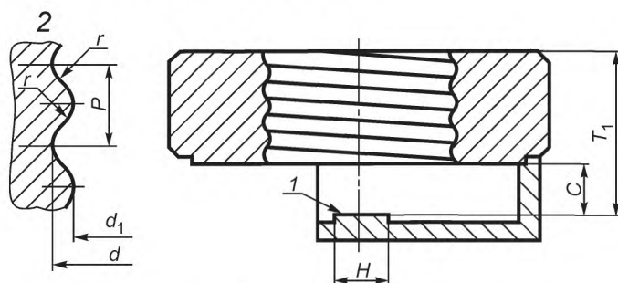
1 — поверхность X; 2 — деталь резьбы (правая резьба)
