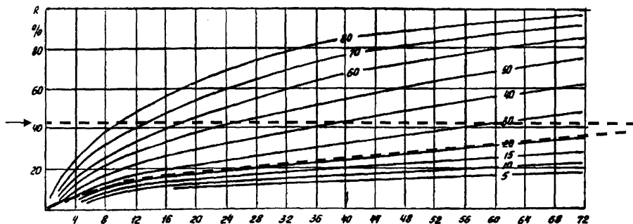
Рисунок П.3. Температурный график
