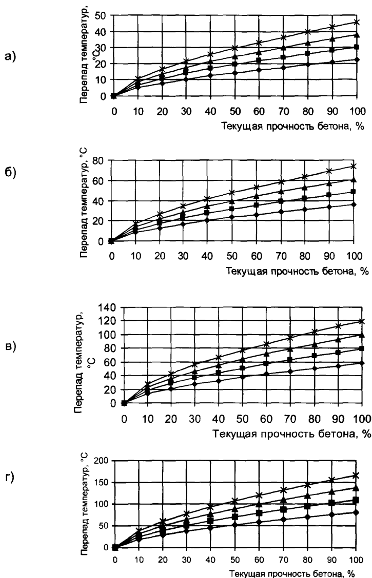
Рисунок 2. Максимальные перепады температур между поверхностью бетона и окружающим воздухом при распалубке
