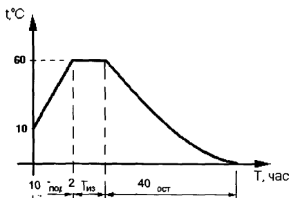
Рисунок П.1. Температурный режим твердения бетона
