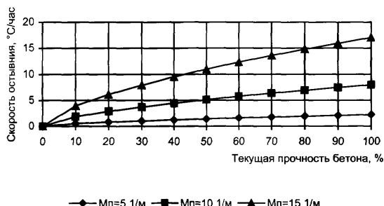
Рисунок 1. Максимальные скорости остывания бетона
