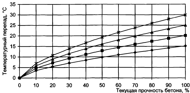
Рисунок 3. Максимальные температурный перепад по сечению конструкции
