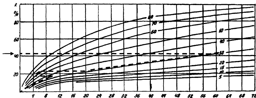
Рисунок П.2. Температурный график
