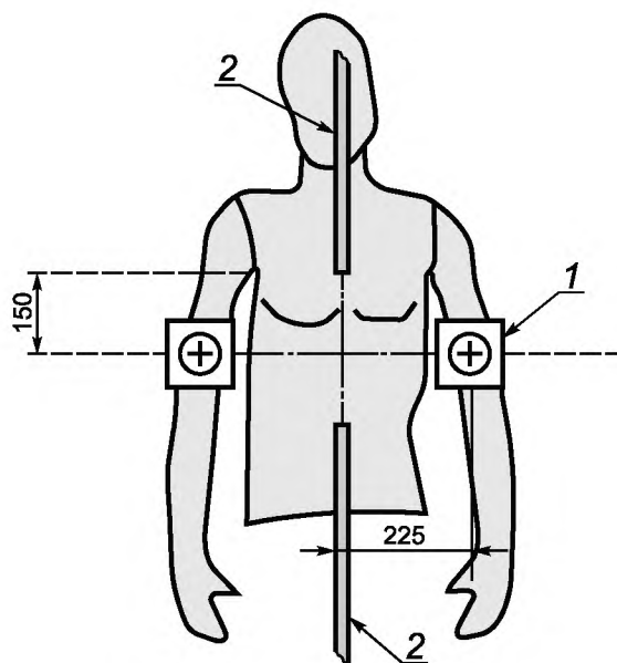
Рисунок 6 – Расположение электродов и контрольных датчиков
