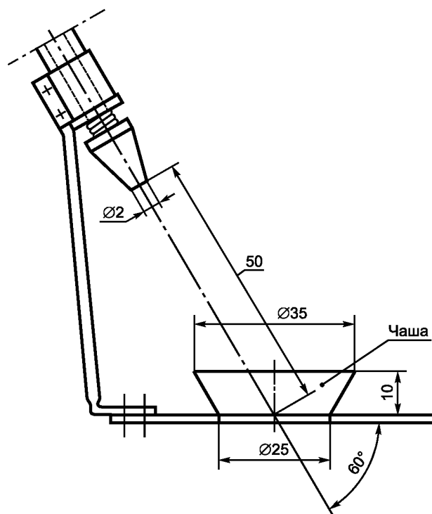
Рисунок 4 — Разбрызгиватель
