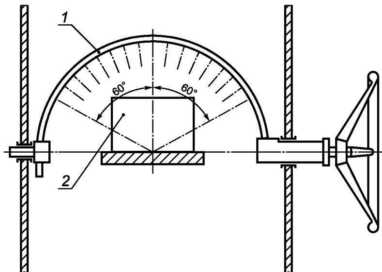
1 — трубка; 2 — образец
