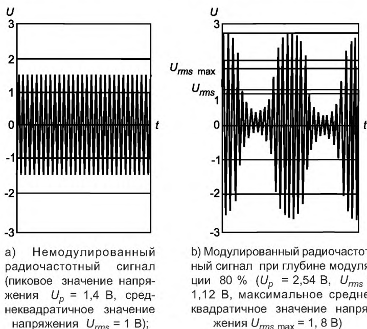
Рисунок 1 – Определение степени жесткости испытаний и формы колебаний на выходе генератора сигналов
