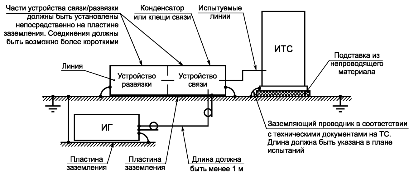
Рисунок 6 — Схема испытаний ТС на устойчивость к НИП
