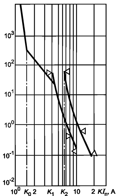
Рисунок 1 — Времятоковые характеристики плавких вставок aM (при любом номинальном токе)
