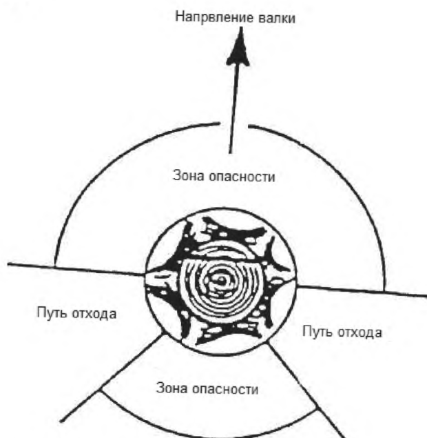
Рисунок ВВ.101 — Описание валки: пути эвакуации
