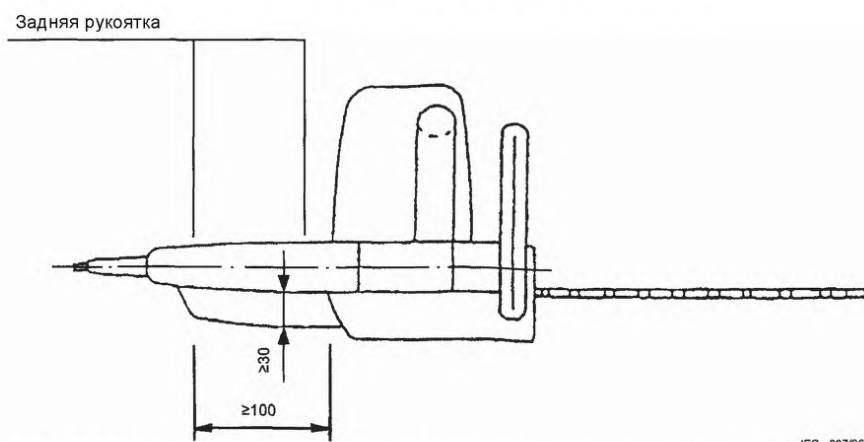
Рисунок 104 — Минимальные размеры (в мм) защитного устройства задней рукоятки
