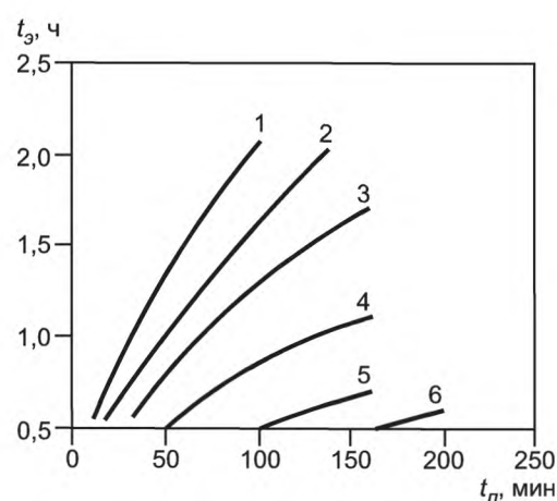
Рисунок Р.4 — Зависимость эквивалентной продолжительности пожара t_3 от продолжительности пожара t_{л} для железобетонных и огнезащищенных металлических конструкций перекрытия при горении ЛВЖ и ГЖ
