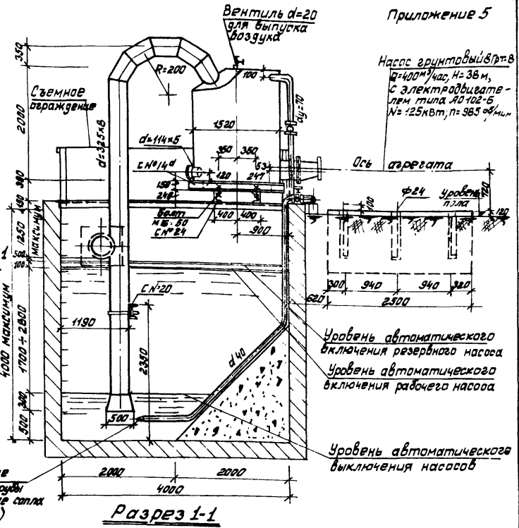
Пример установки насосов с вакуумными баками
