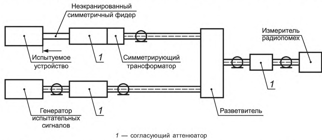
Рисунок 8 — Структурная схема измерения напряжения ИРП на симметричном антенном входе
