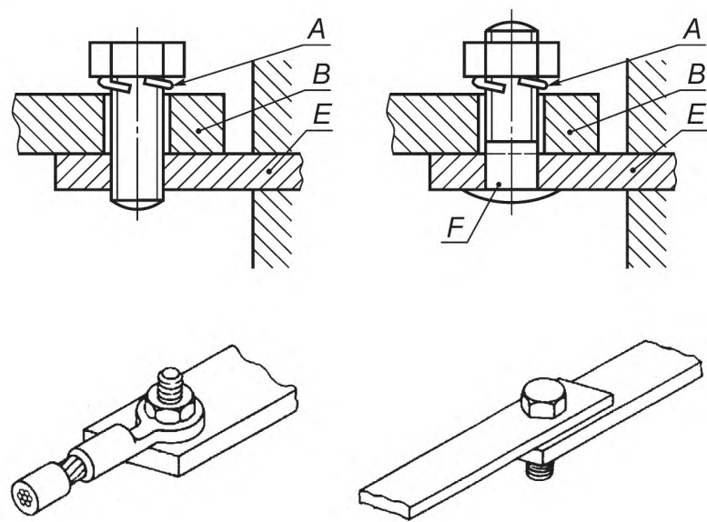
A — запорное устройство; B — кабельный наконечник или шина; E — неподвижная часть; F — штифт
