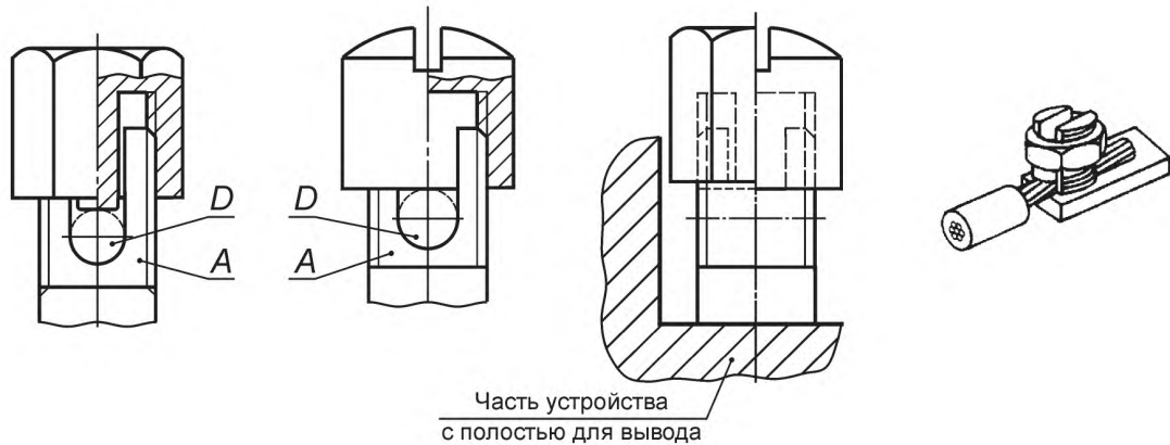
A — неподвижная часть; D — место для проводника
