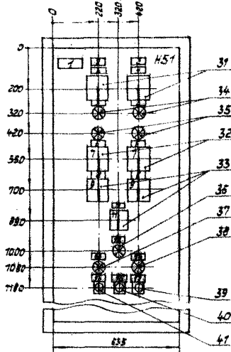
Вид сверху М150
