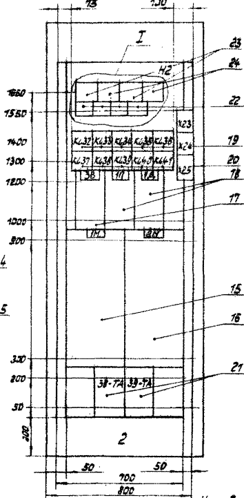
Вид спереди (вторая сторона) Дверь не показана
