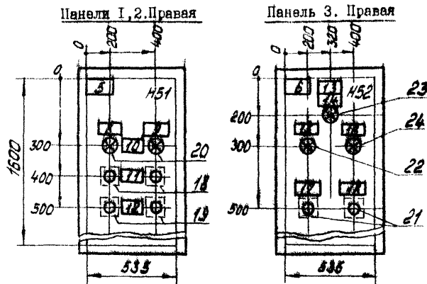
Двери щита
