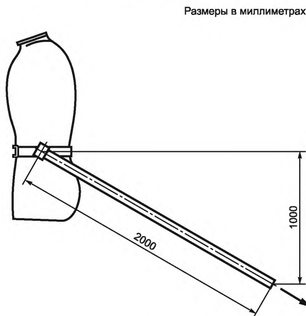
Рисунок 4 — Схема испытания прочности ремennого крепления к туловищу или ремня шланга подачи воздуха
