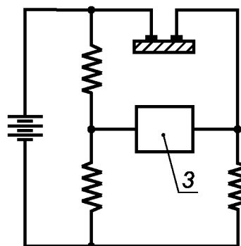
б) Метод моста Уитстона
