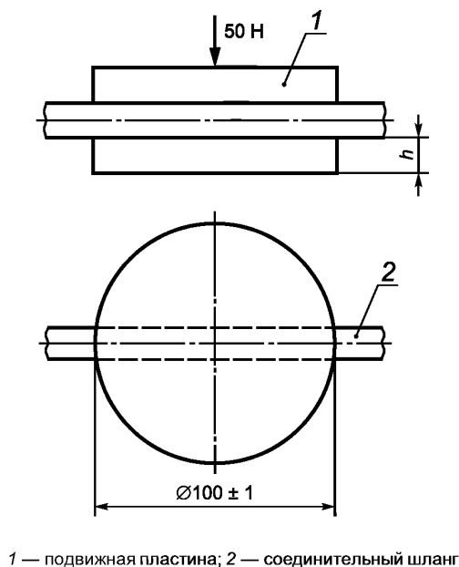
Рисунок 1 — Схема испытания
