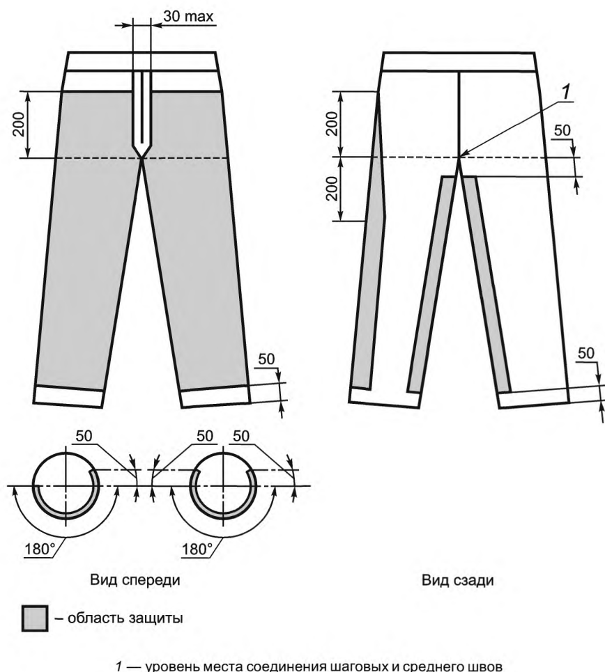
Рисунок 2 — Конструкция В
