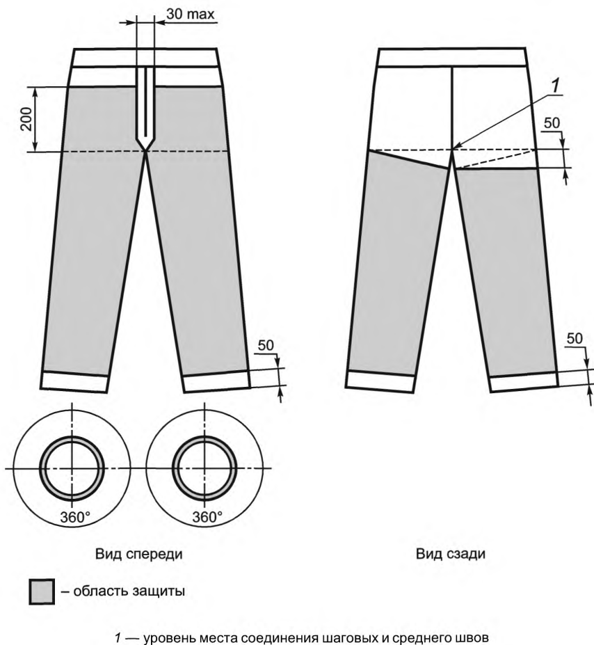
Рисунок 3 — Конструкция С
