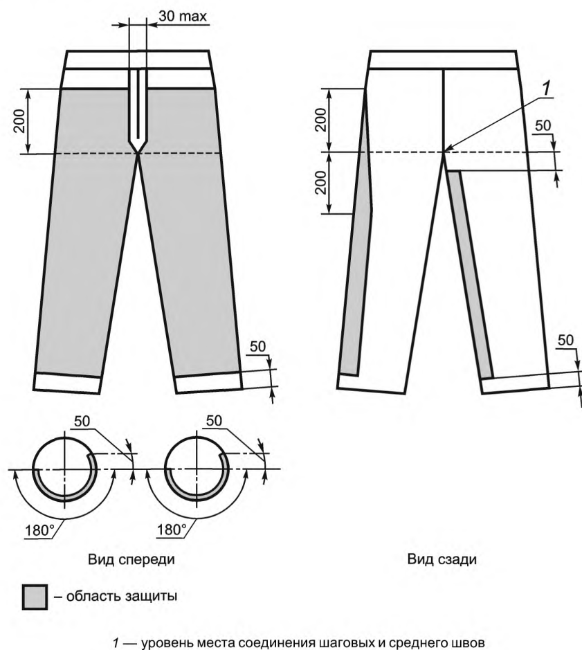
Рисунок 1 — Конструкция А
