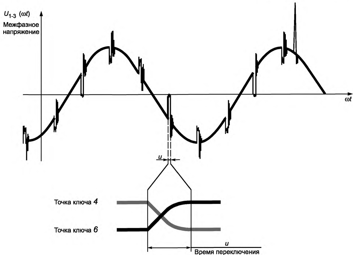
Рисунок В.13 — Провалы при коммутации в схемах с трехфазным 6-пульсным мостовым преобразователем
