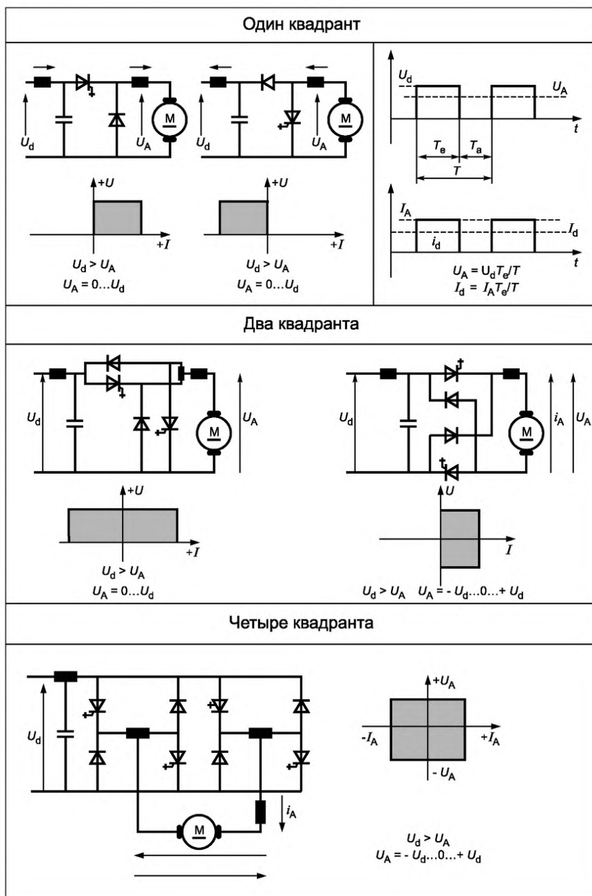
Рисунок F.2 — Преобразователи с внутренней коммутацией (прерыватели)
