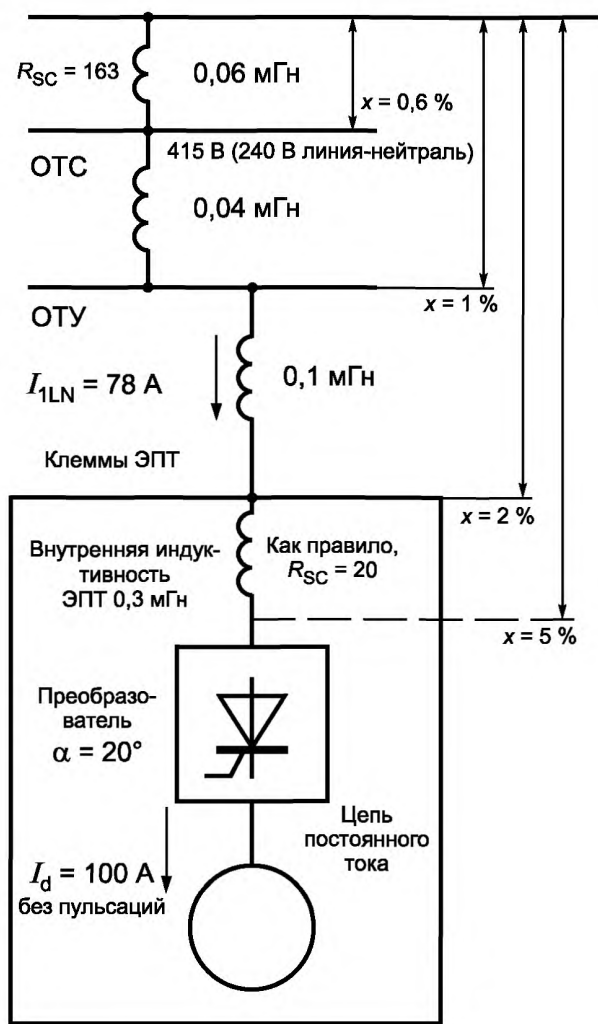
Рисунок В.11 — Пример простой структуры
