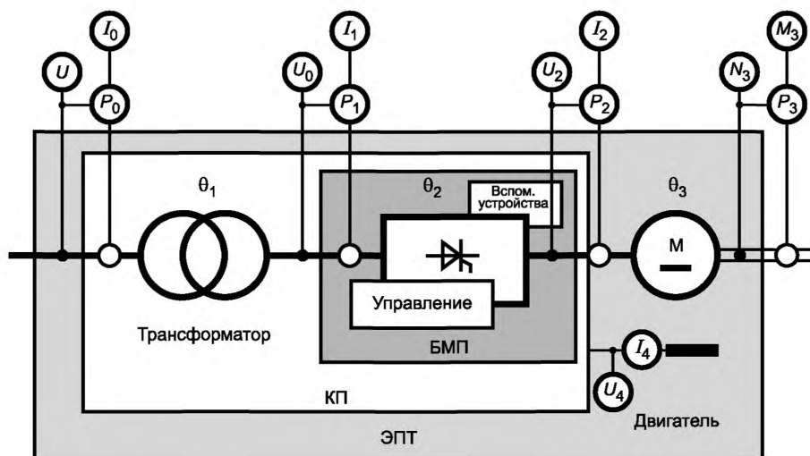
Рисунок 7 — Схема испытаний ЭПТ
