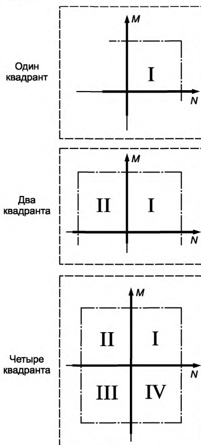
Рисунок 3 — Рабочие квадранты работы электропривода
