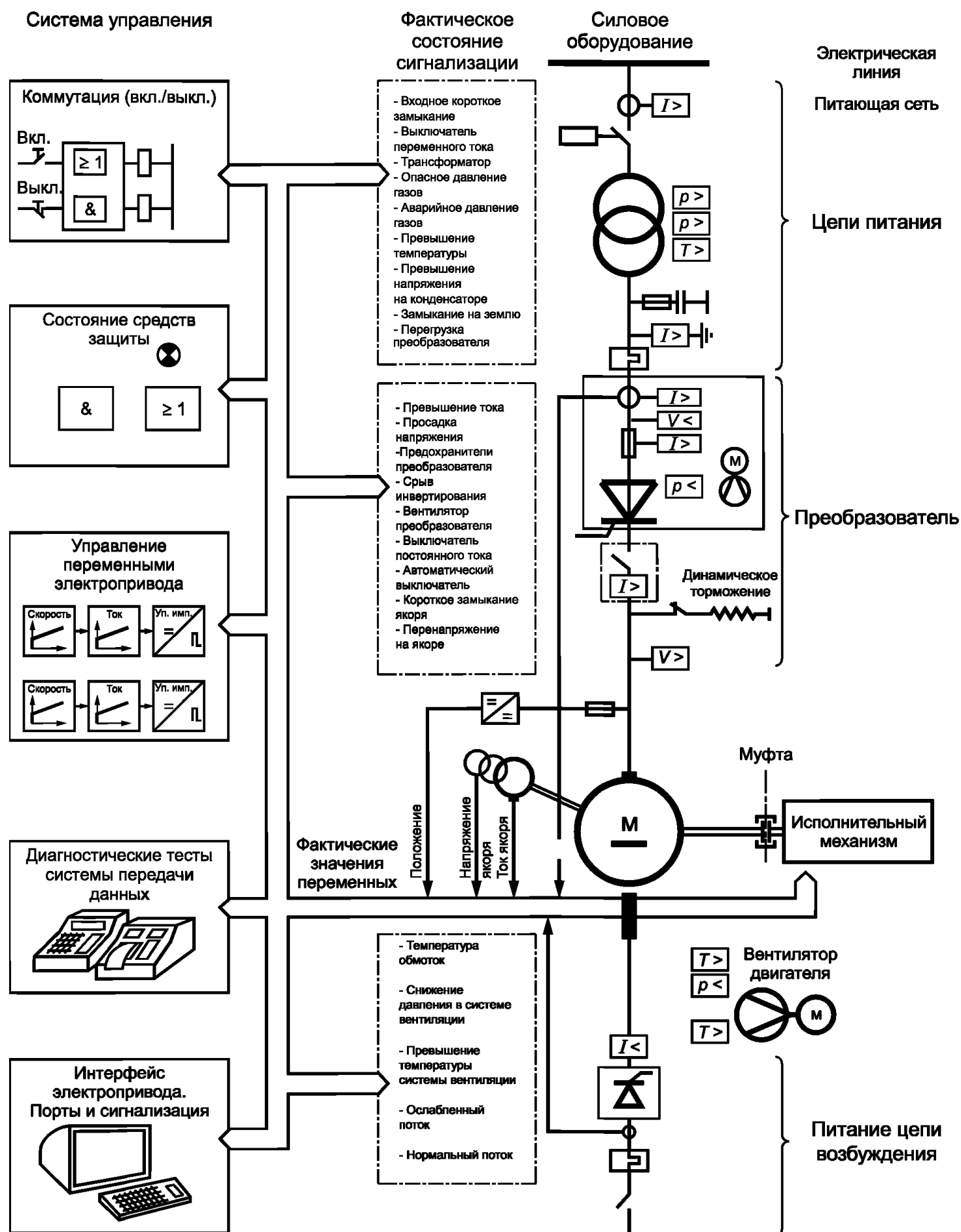
Рисунок 1 — Функциональная схема электропривода постоянного тока
