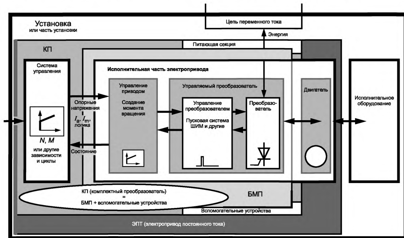
Рисунок D.8 — Структура системы электропривода
