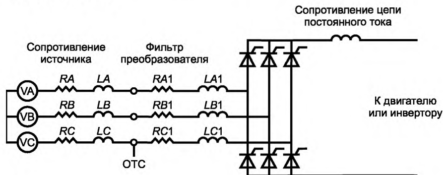
Рисунок В.1 — Тиристорный преобразователь с большой индуктивностью в цепи постоянного тока
