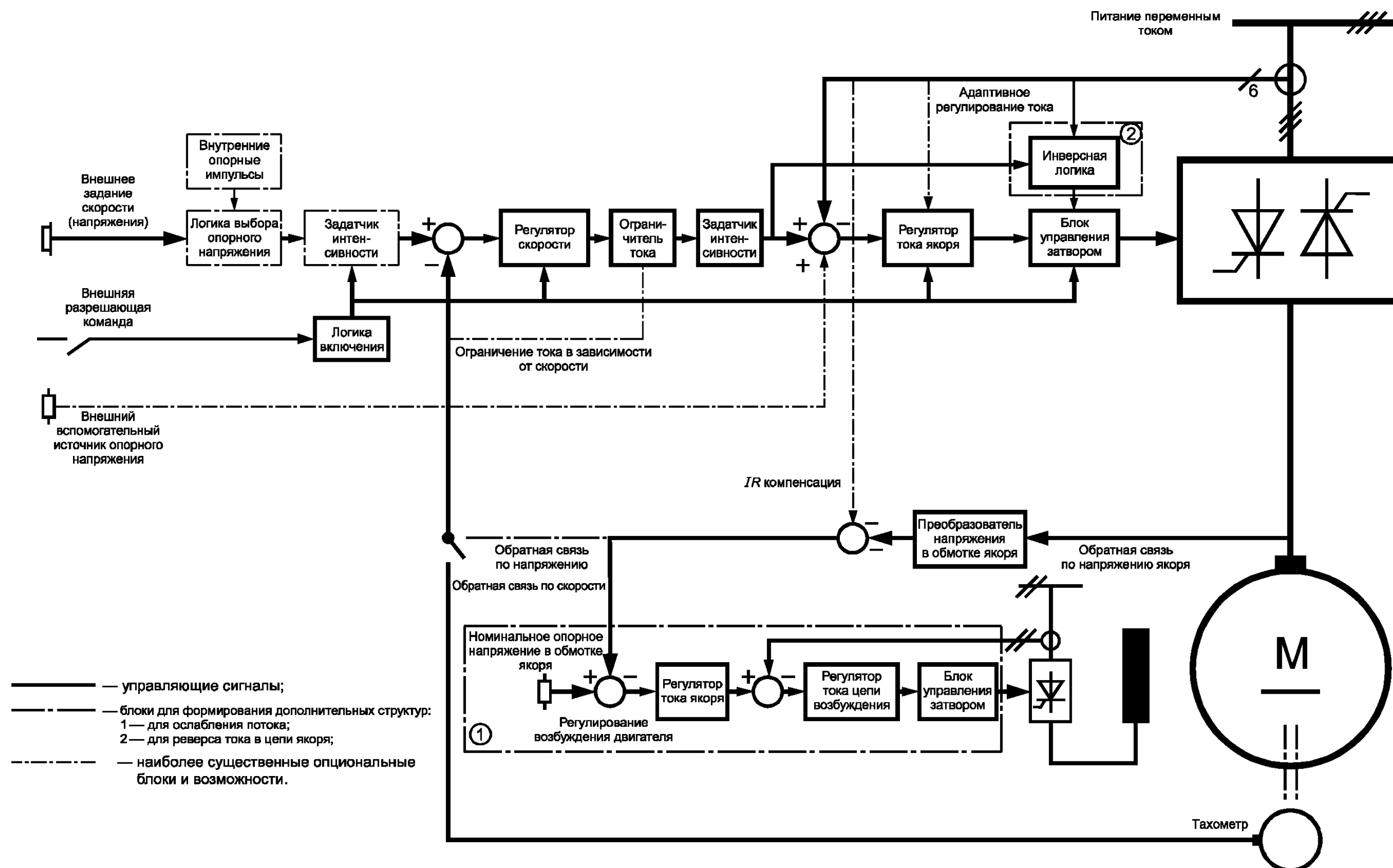
Рисунок D.2 — Блок-схема
