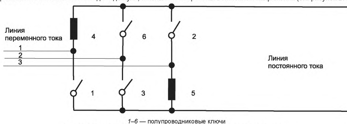
Рисунок В.12 – Трехфазный 6-пульсный мостовой преобразователь
