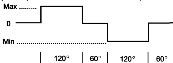
Рисунок 4 — Квазипрямоугольные колебания
