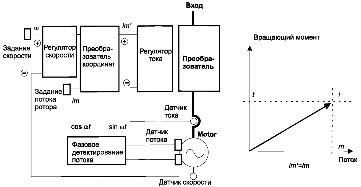
Рисунок D.6 – Векторное управление со слежением за полем (инвертор – источник напряжения)
