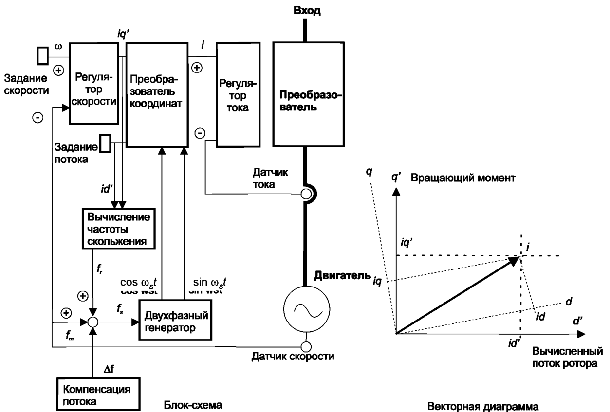
Рисунок D.7 – Векторное управление с вычислением частоты скольжения (инвертор – источник напряжения)
