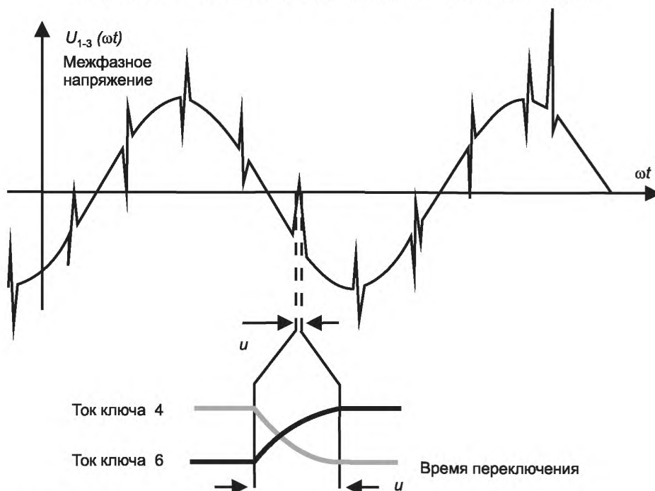
Рисунок В.12 – Трехфазный 6-пульсный мостовой преобразователь
