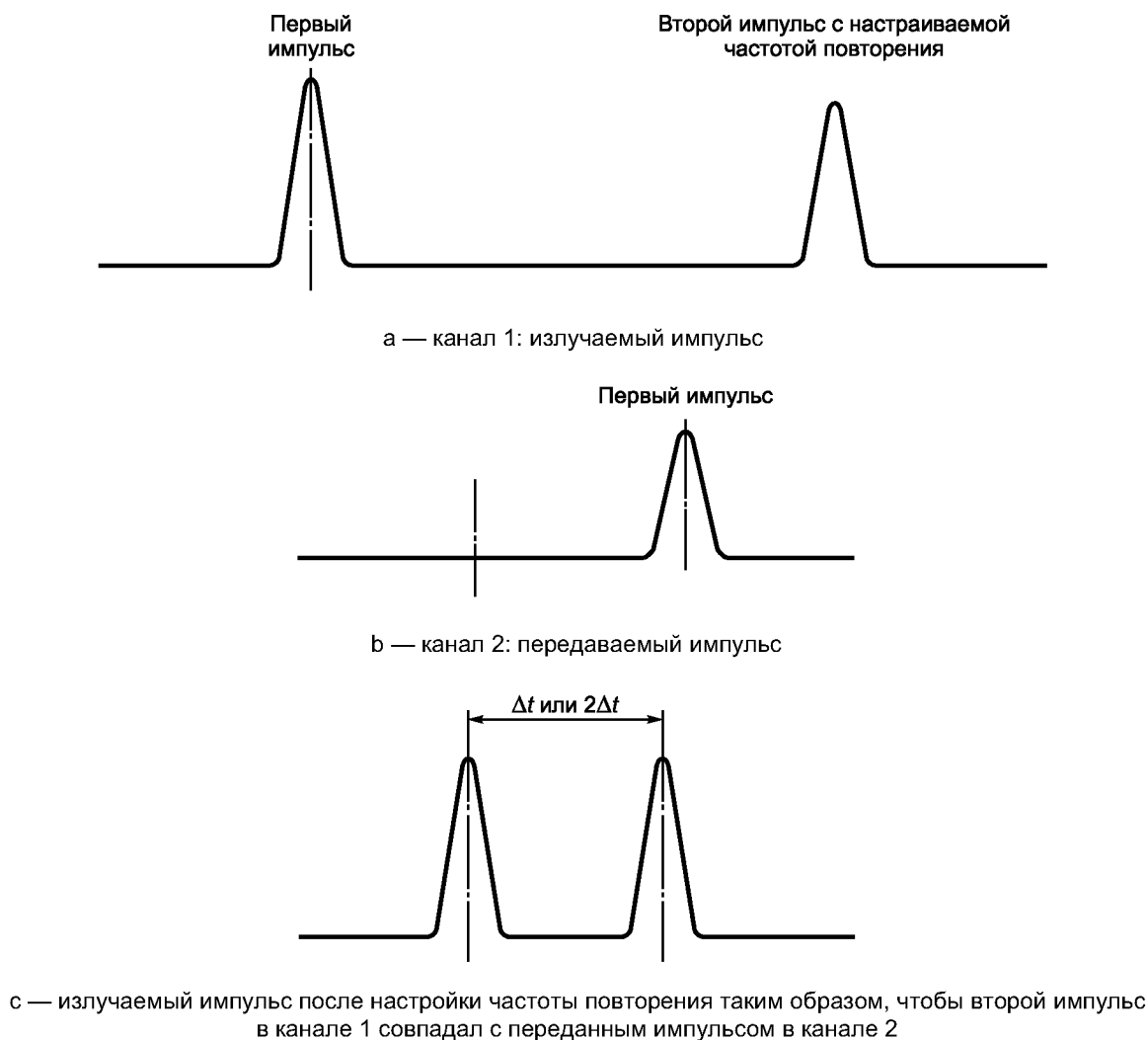
Рисунок А.3 — Принцип измерения длины волокна
