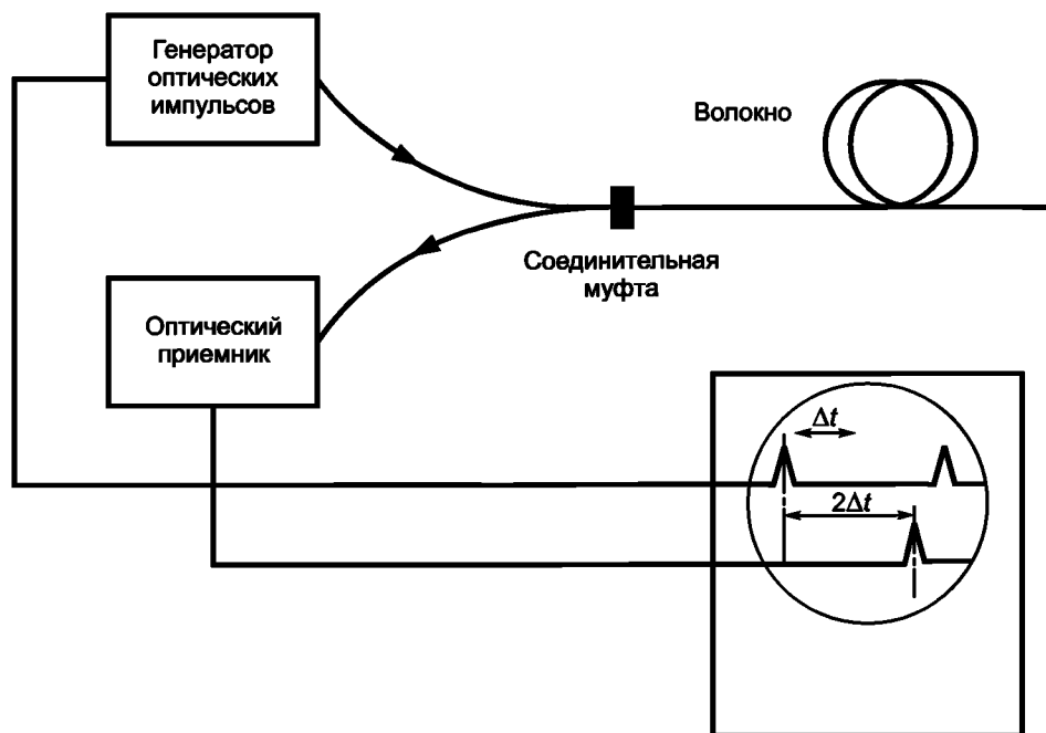
Рисунок А.2 — Измерение времени задержки отраженного импульса
