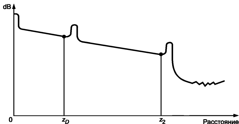
Рисунок В.5 — Схематическая линия OPBO образца (от z_D до z_2 ) с секцией кабеля (например, компенсирующей катушкой с волокном) известной длины z_D , предшествующей ему (метод одной точки по В.4.3.3)
