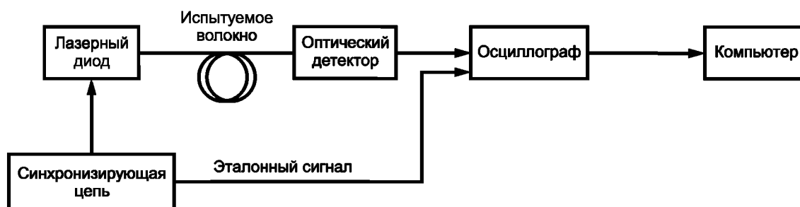
Рисунок С.2 — Расположение оборудования для метода дифференциальной задержки импульса (см. С.2.2.2)
