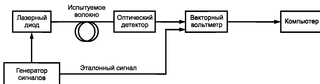
Рисунок С.1 — Расположение оборудования для метода фазового сдвига (см. С.2.2.1)
