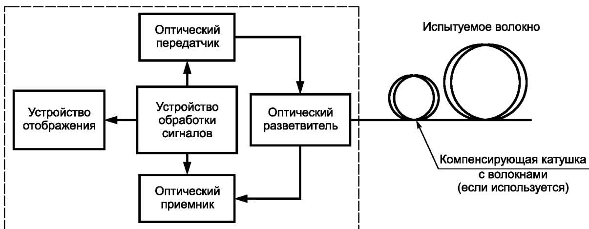
Рисунок В.1 — Блок-схема ОРВО
