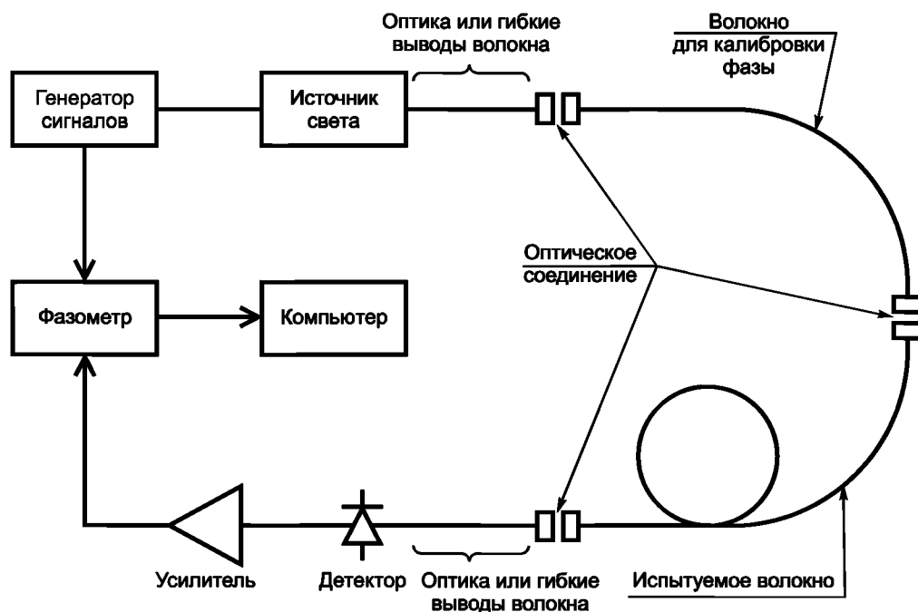
Рисунок Е.1 — Оборудование для измерения длины волокна
