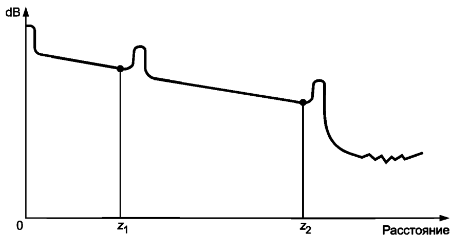
Рисунок В.3 — Схематичная линия ОРВО образца (от z_1 до z_2 ) с секцией кабеля (например, компенсирующей катушкой с волокном) неизвестной длины z_1 , предшествующей ему, и с импульсом отражения от точки соединения волокна (метод двух точек по В.4.3.1)
