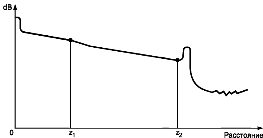
Рисунок В.2 — Схематическая линия ОРВО образца (от z_1 до z_2 ) с секцией кабеля (например, компенсирующей катушкой с волокном) неизвестной длины z_1 , предшествующей ему, и без импульса отражения от точки соединения волокна (метод двух точек по В.4.3.1)
