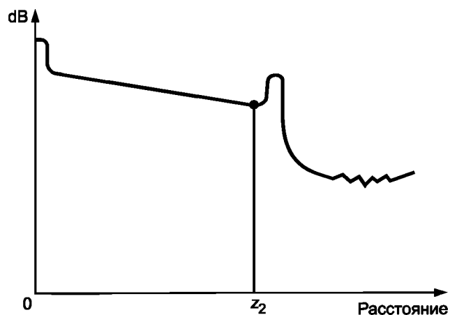
Рисунок В.4 — Схематичная линия ОРВО образца (от 0 до z_2 ) без секции кабеля, предшествующей ему (метод одной точки по В.4.3.2)
