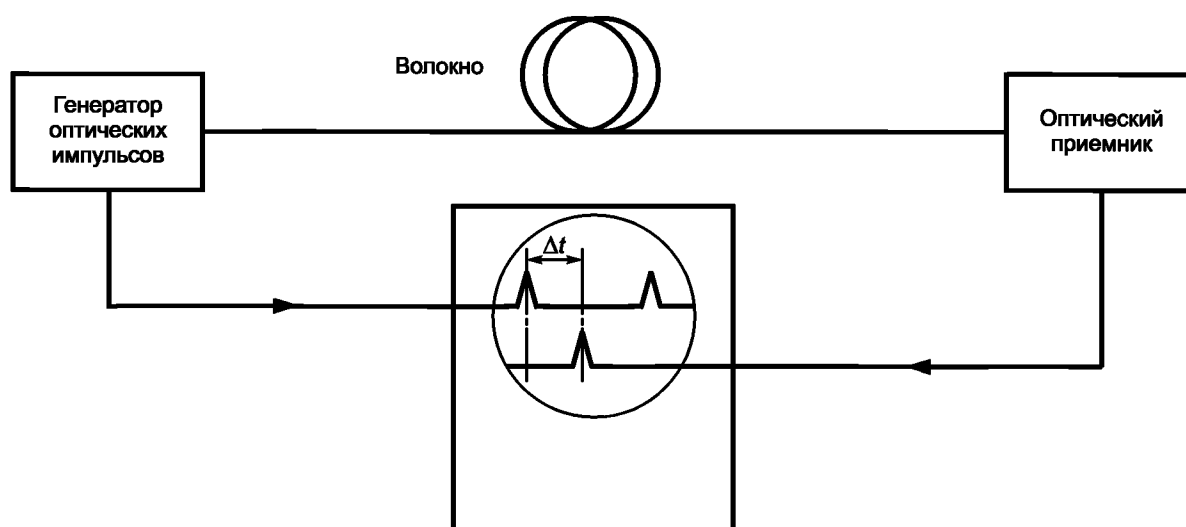
Рисунок А.1 — Измерение времени задержки прохождения оптического импульса
