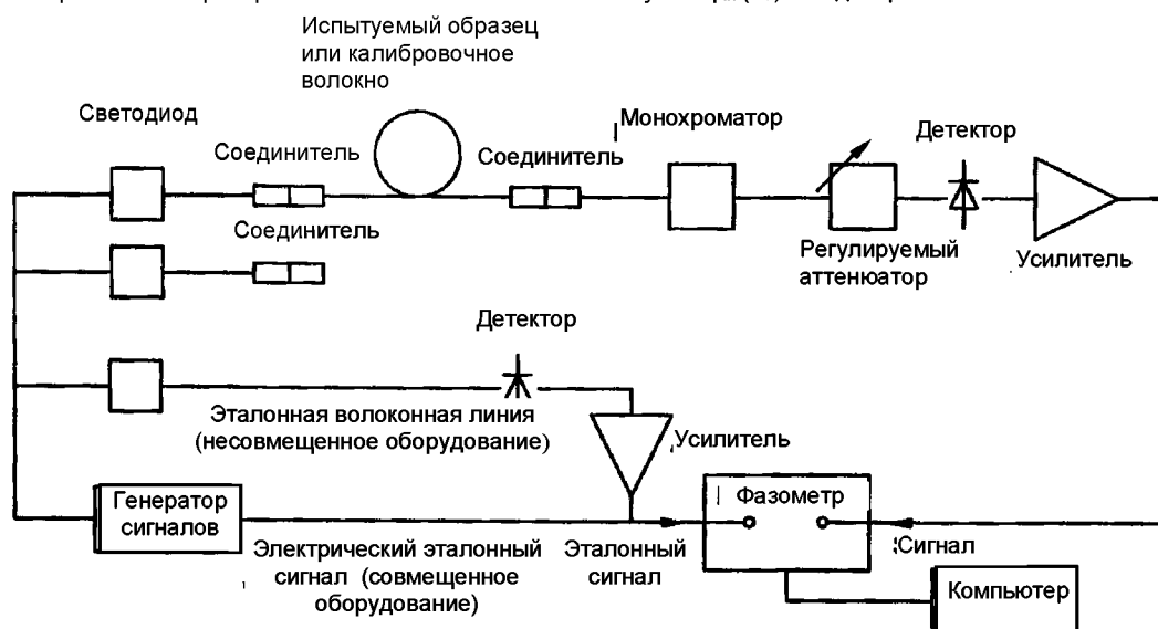
Рисунок А.3 – Комплект оборудования для измерения хроматической дисперсии. Система на основе светодиодов (типовая)
