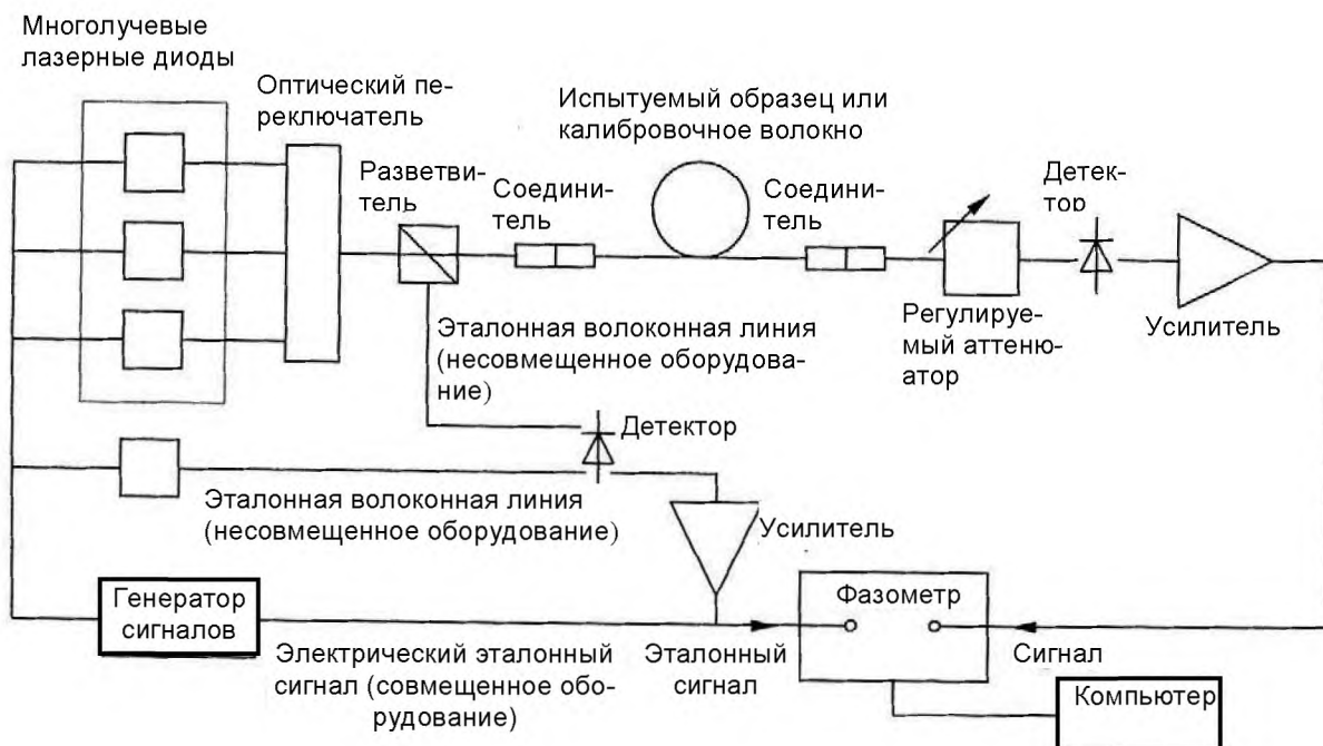
Рисунок А.1 – Комплект оборудования для измерения хроматической дисперсии. Система на основе многолучевого лазера (типичная)
