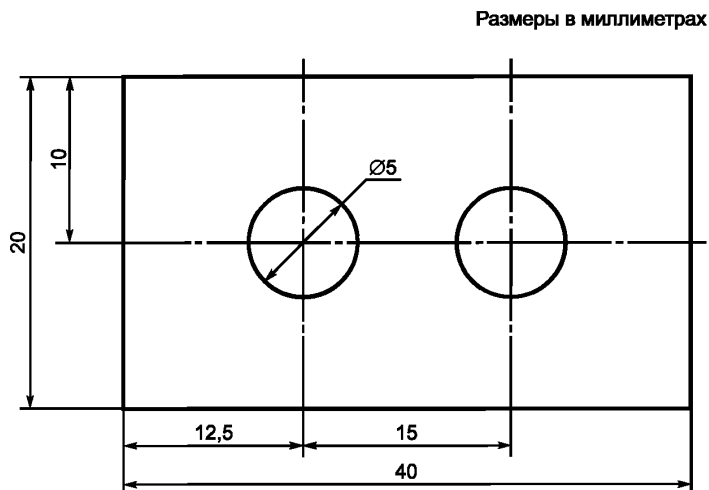
Рисунок 35 — Образец для проведения испытаний на сопротивление изоляции
