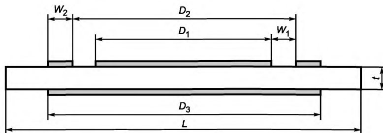
Рисунок 24 — Электроды для измерений объемного и поверхностного сопротивления
