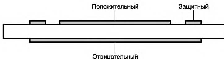
Рисунок 22 — Измерение объемного сопротивления
