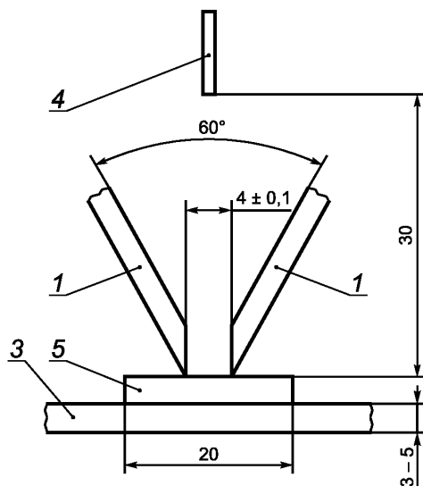
1 — электрод платиновый; 3 — опора (стеклянная); 4 — источник капель; 5 — образец
