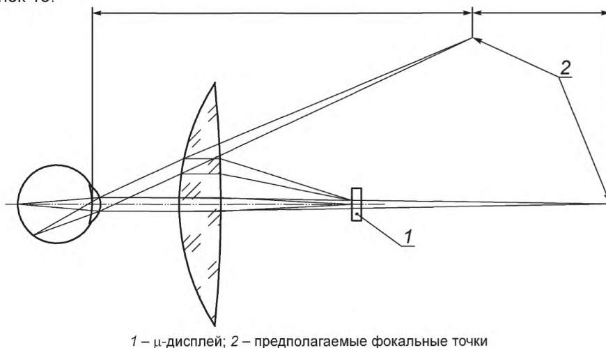
Рисунок 15 – Фокусное расстояние
