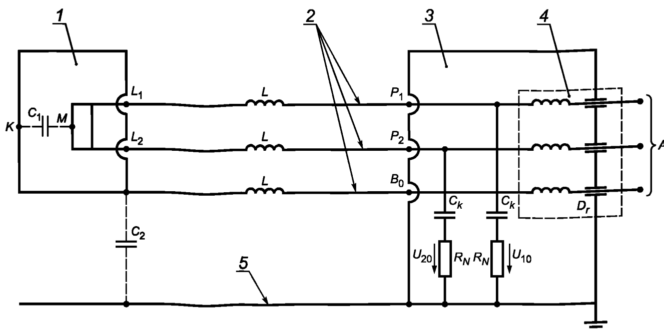
а) Схема измерения и схема питания
