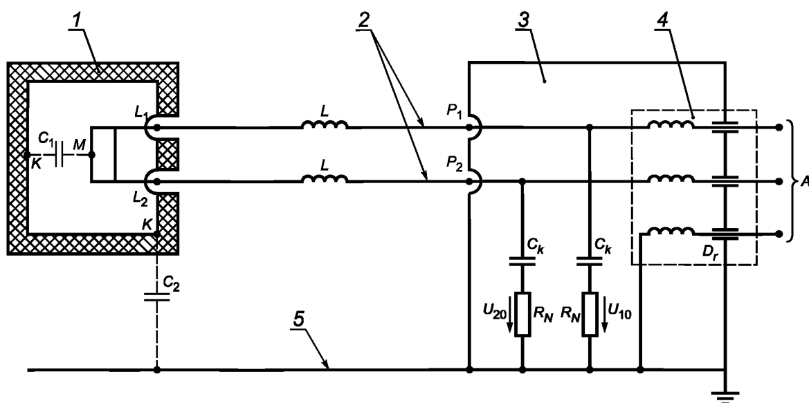
а) Схема измерения и схема питания
