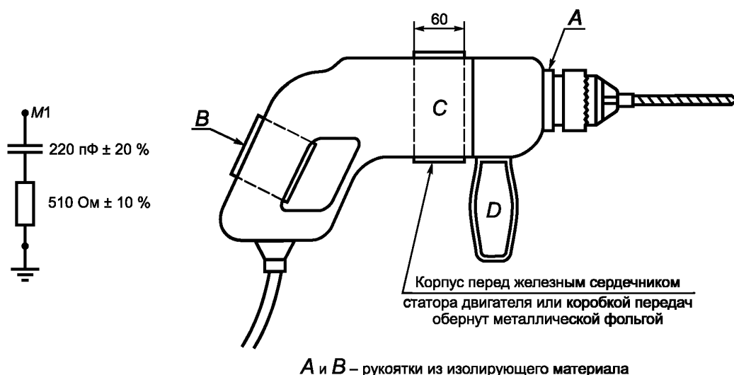
Рисунок 12 — Элемент RC для эквивалента руки (см. 7.4.2.3)
