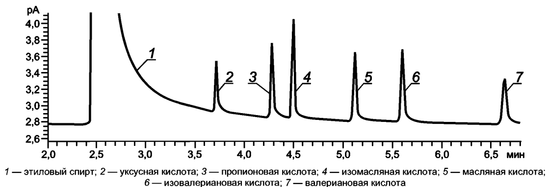
Рисунок 1 — Хроматограмма анализа градуировочной смеси на содержание летучих кислот
