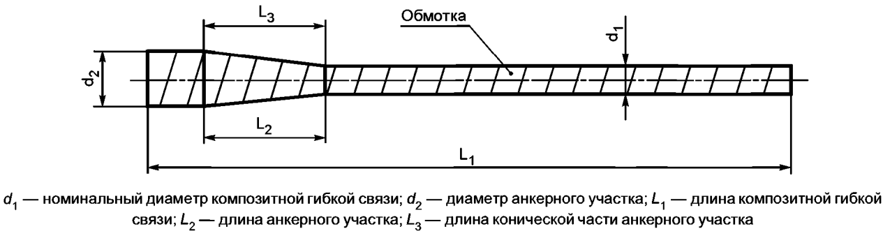
Рисунок Л.1 — Композитная гибкая связь с выделенным цилиндроконическим анкерным участком
