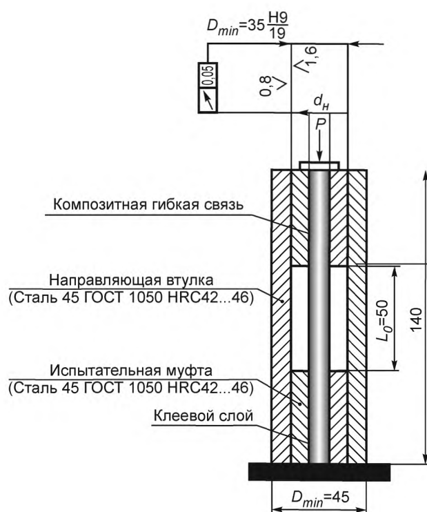
Рисунок В.1 — Конструкция приспособления для испытания образцов
