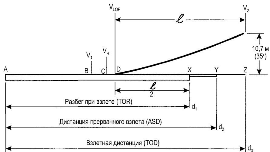
а) С неработающими двигателями
