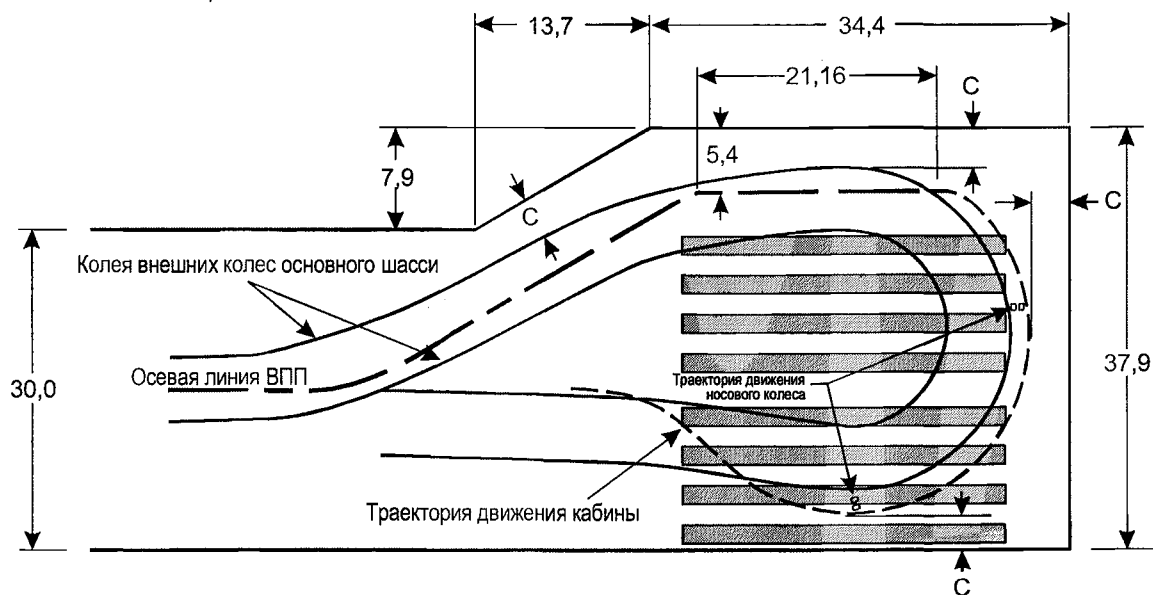
Рис. А4-3. Схема площадки разворота на ВПП для воздушных судов, обозначенных кодовой буквой В
