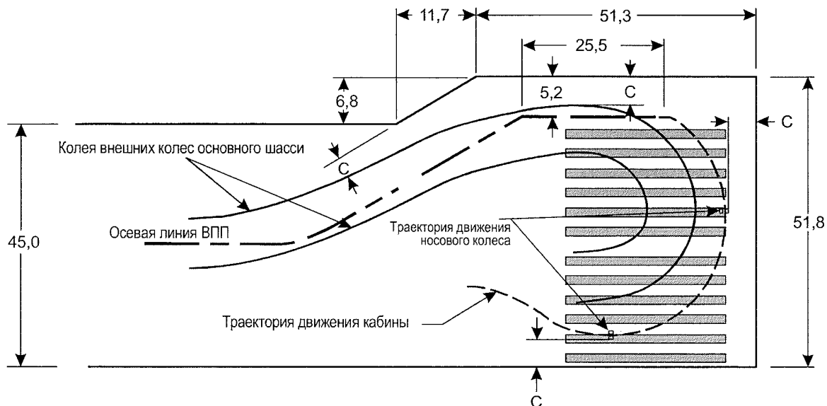
Рис. А4-4. Схема площадки разворота на ВПП для воздушных судов, обозначенных кодовой буквой С
