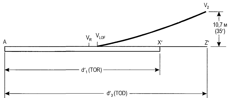
б) Со всеми работающими двигателями
