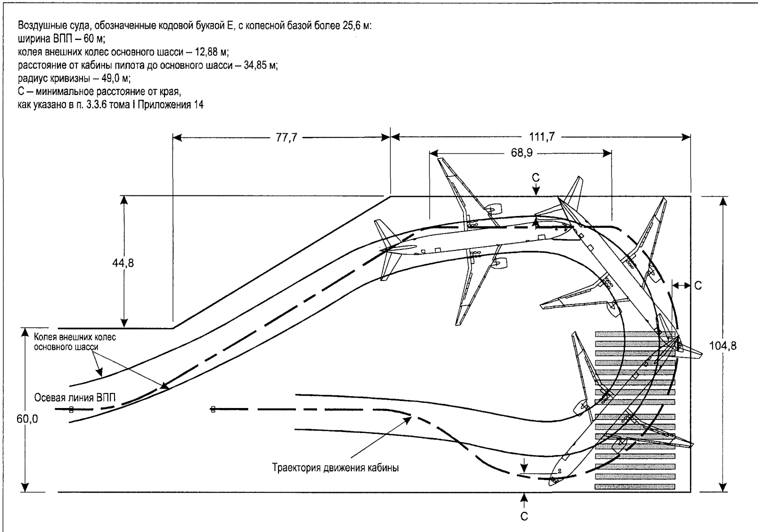
Рис. А4-9. Схема площадки разворота на ВПП для воздушных судов, обозначенных кодовой буквой Е (колесная база более 25,6 м; ширина ВПП – 60 м)
