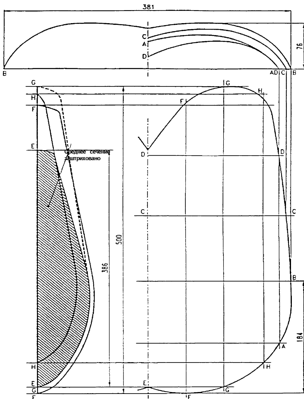
Рисунок А.2 — Размеры нагрузочного штампа для сиденья, прессованного из стекловолокна
