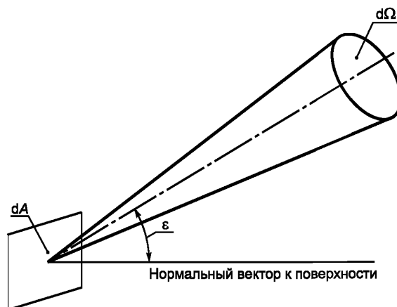
Рисунок 2 — Определение энергетической яркости
