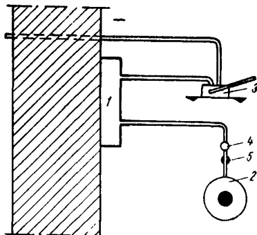
Рис. 10. Принципиальная схема установки для исследования воздухопроницаемости стыка в натуральных условиях
