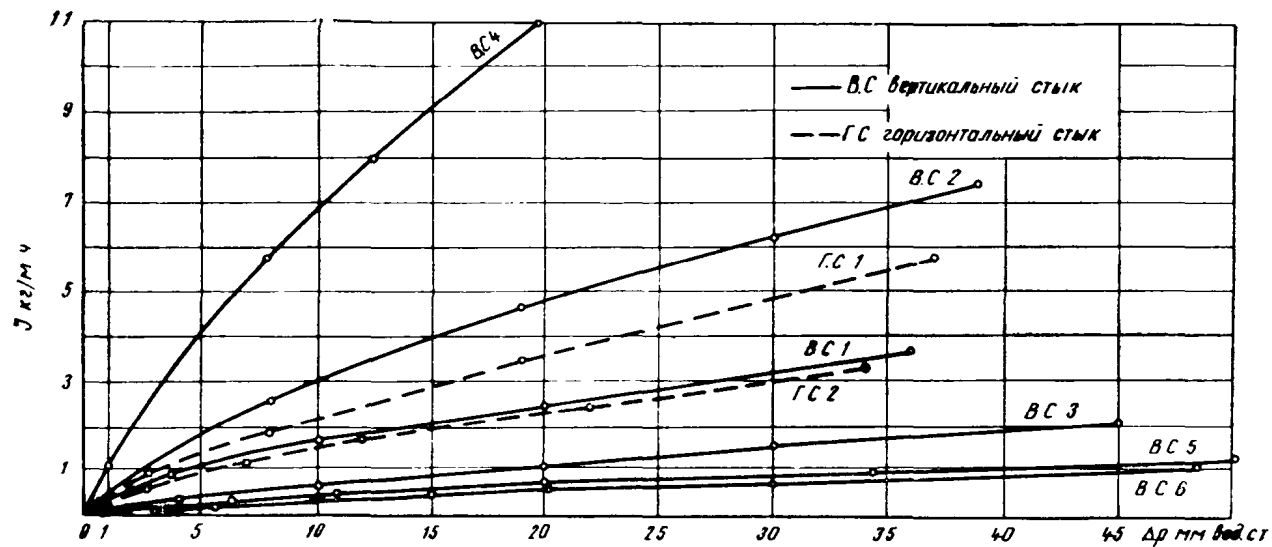
Рис. 11. Кривая воздухопроницаемости стыка
