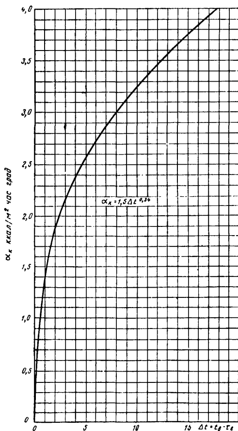
Рис. 6. График для определения \alpha_k у вертикальных поверхностей
