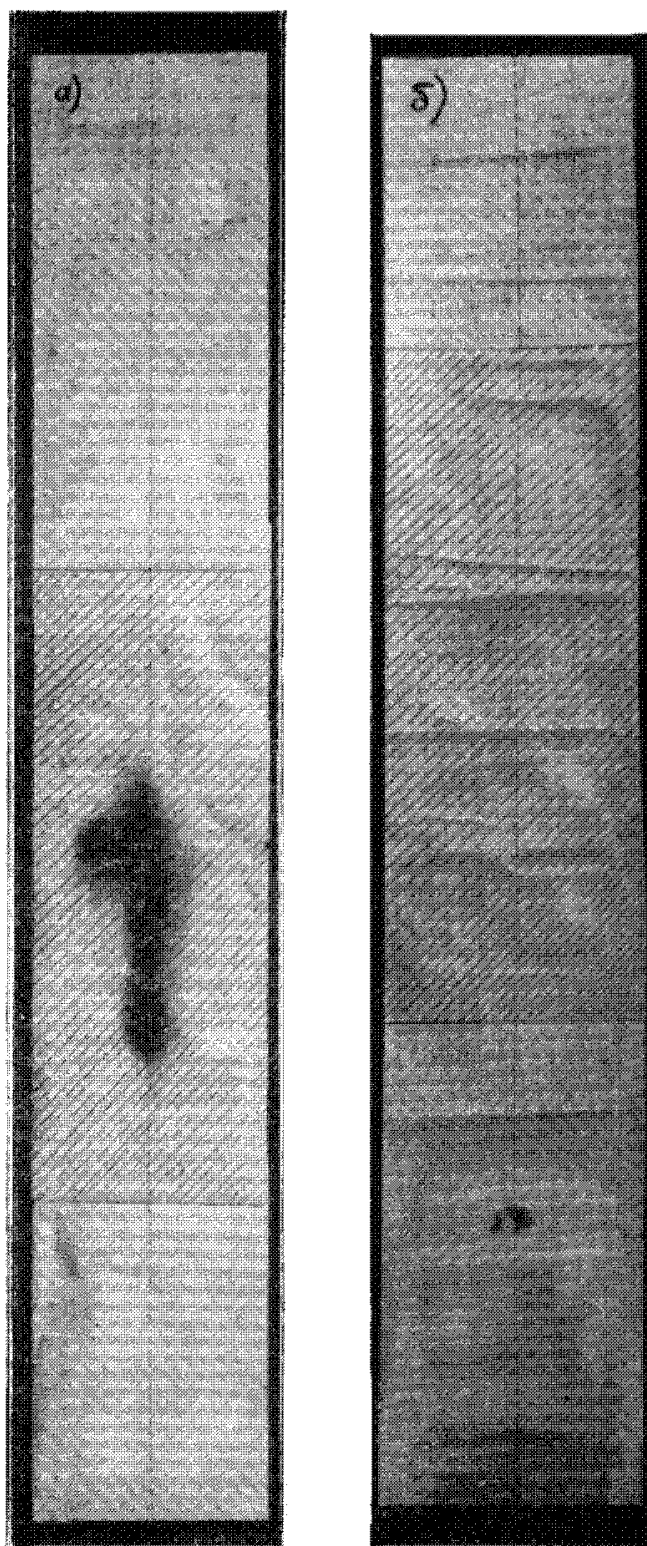
Рис. 12. Окраска светочувствительной бумаги при испытании стыка химическим методом
