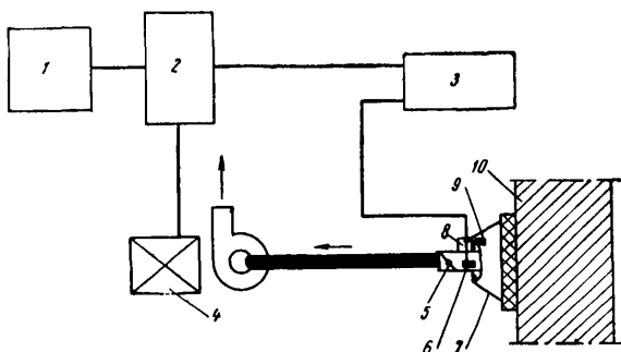
Рис. 13. Принципиальная схема прибора ИВС-1
