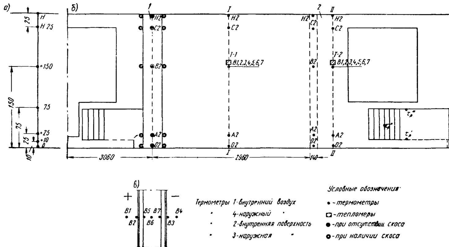
Рис. 1. Размещение датчиков при проведении проверки в зимних и летних условиях а — центральная вертикаль; б — развертка стен; в — сечение стены; 1 — наружный угол со скосом; 2 — стык
