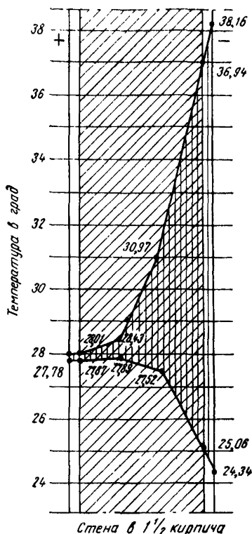
Рис. 9. График затухания температурных колебаний в толще стены
