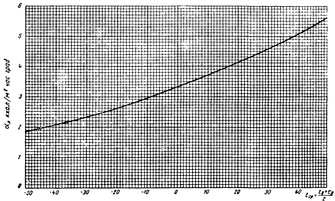
Рис. 7. График для определения \alpha_1 у вертикальных поверхностей
