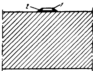
Рис. 3. Установка датчиков на поверхности ограждения 1 — термометр; 2 — гипс
