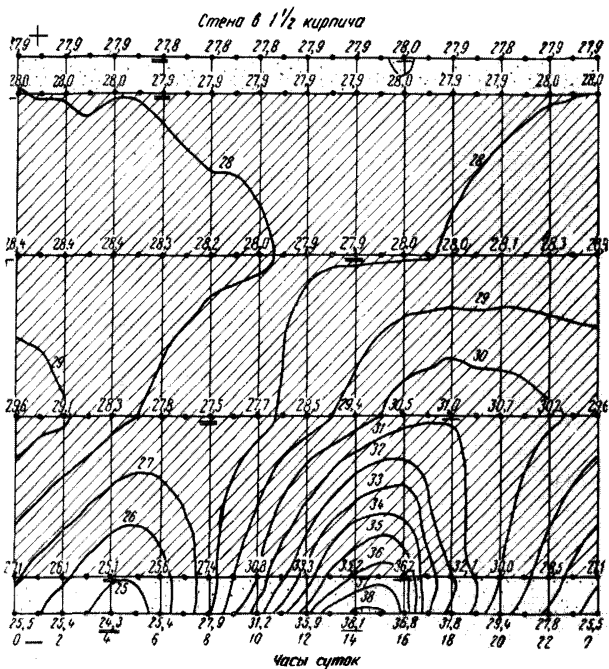
Рис. 8. Термоизоплеты (изотермы во времени)
