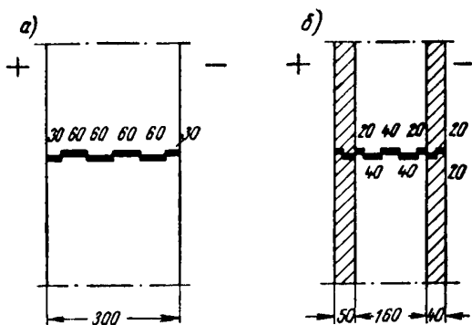
Рис. 5. Примерные схемы отбора проб из панелей
