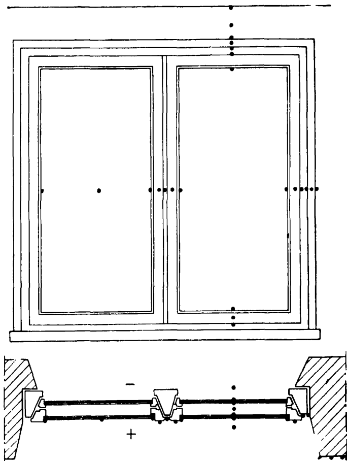
Рис. 2. Размещение датчиков на внутренней поверхности окна
