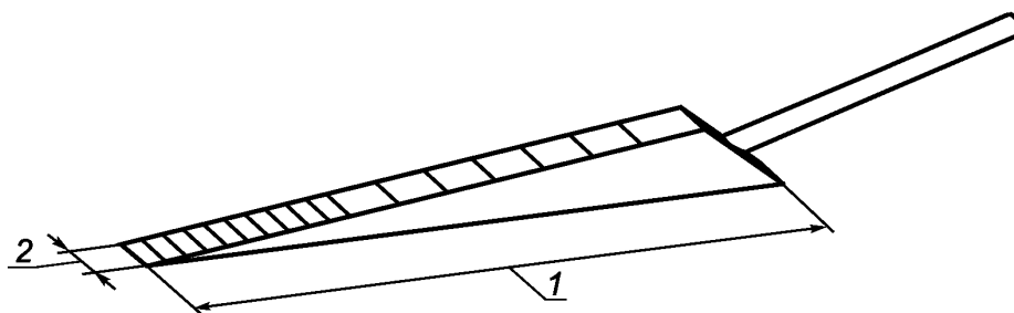
1 — длина (300 \pm 1) мм; 2 — ширина (25 \pm 1) мм
