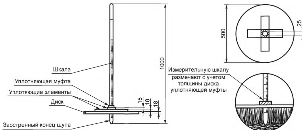
Рисунок 2 — Измерительный диск
