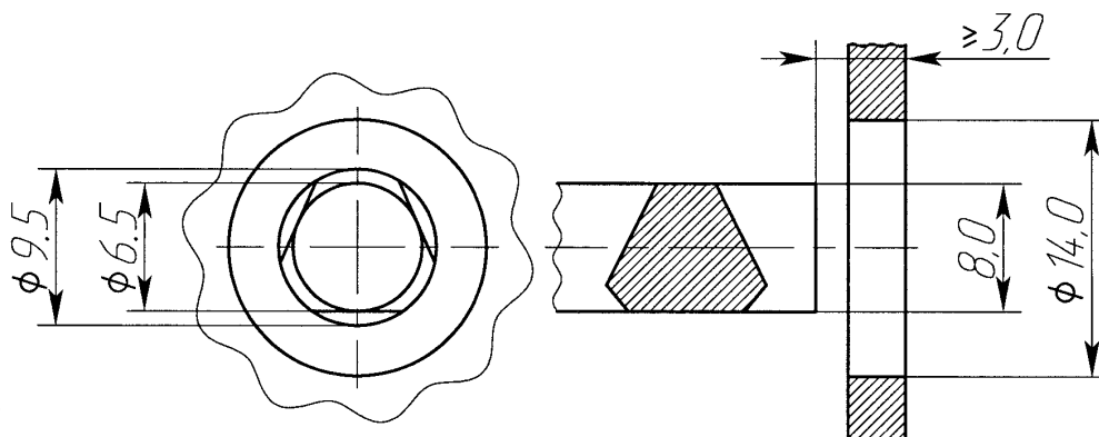
Рисунок 9 - Треугольный ключ для запирания двери по ГОСТ Р 53780
