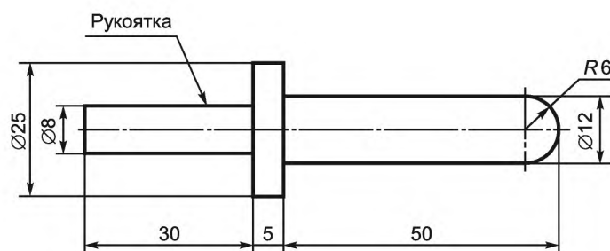
Рисунок 103 — Испытательный щуп
