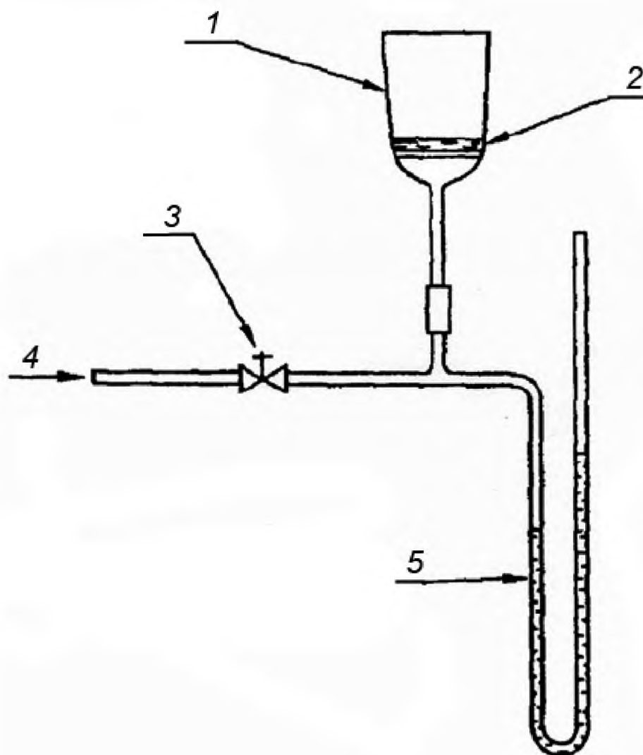
1 — воронка с фильтром из спеченного стекла; 2 — испытуемая жидкость; 3 — тонко регулируемый клапан; 4 — подача отфильтрованного воздуха; 5 — манометр
