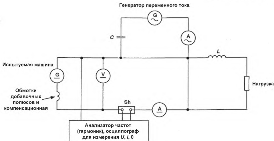
Рисунок 1 – Определение индуктивности цепи якоря с учетом насыщения
