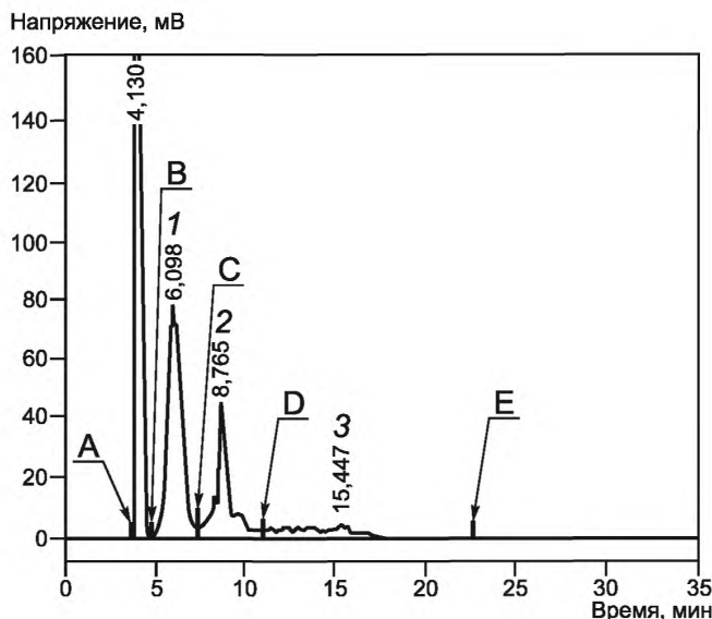
Рисунок 4 — Хроматограмма с идентифицированными пиками и изображенной интеграцией
