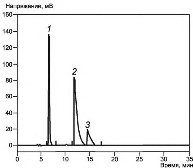
Рисунок 3 — Хроматограмма калибровочного раствора А
