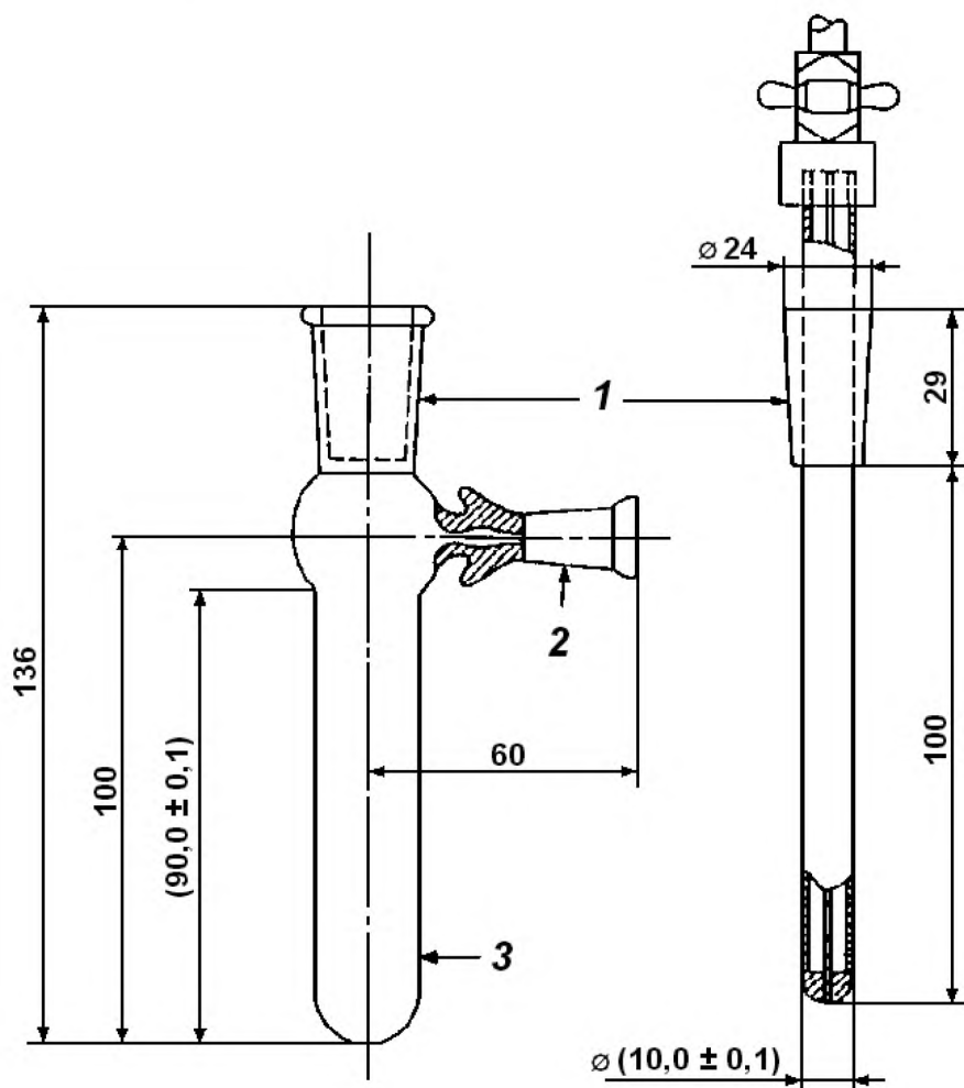
1 — конусное соединение 24/29 (по стандарту [3]); 2 — конусное соединение 10/19 (по стандарту [3]); 3 — трубка наружным диаметром (18,0 \pm 0,2) мм и внутренним диаметром (16,0 \pm 0,2) мм (по стандарту [1])
