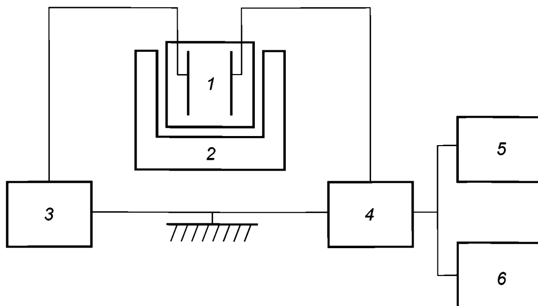
1 — испытательная камера; 2 — нагревательное устройство; 3 — генератор прямоугольного сигнала; 4 — измерительная цепь; 5 — измерительный прибор; 6 — записывающее устройство
