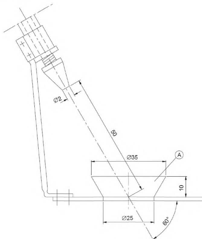
Рисунок 101 – Устройство для испытания обрызгиванием
