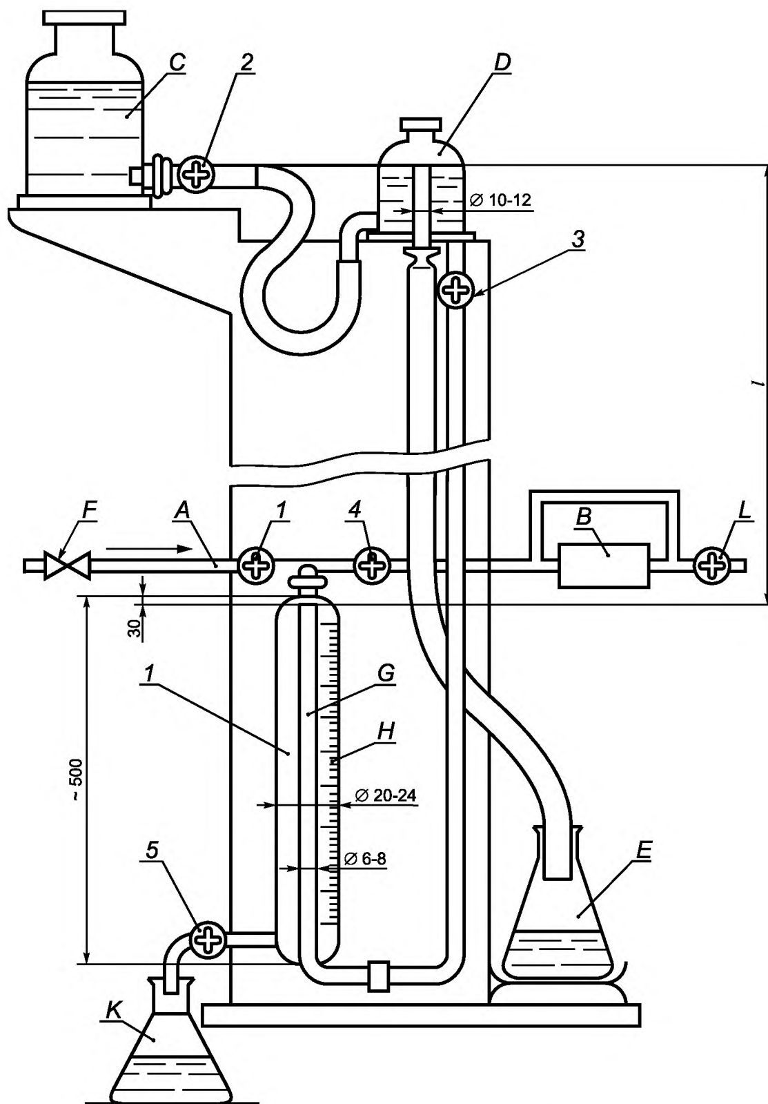
\ell — расстояние между уровнем воды в сосуде линии изгиба трубки; А — вход; В — испытуемый образец; С — емкость с водой; D — сосуд с постоянным уровнем воды; E, K — переливные сосуды; F — регулятор; G — трубка; H — измерительная бюретка; L — выход клапана; 1—5 — ручные краны
