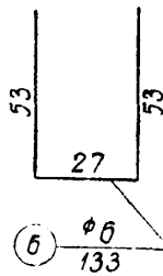
№ стержней Диаметр мм Длина см Количе- ство шт. Общая длина м Объем бетона и содержание арматуры 1 22 704 24 169,0 Бетона—20,6 м³ 2 22 817 16 130,7 3 22 732 16 116,5 4 22 624 8 49,9 5 8 644 60 386,0 6 6 133 272 362,0 Арматуры — 118 кг/м³ 7 12 1039 36 374,0 8 12 236 114 269,0 9 12 242 99 240,0 10 6 126 54 68,0
