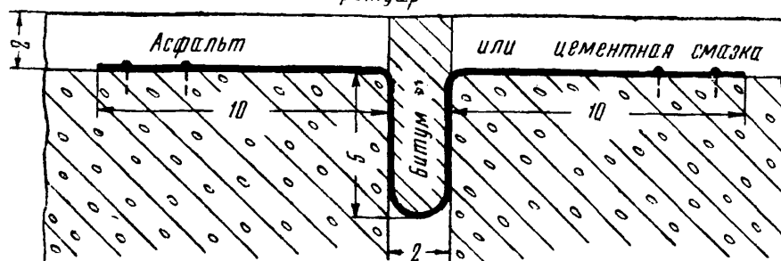
Б Тротуар
