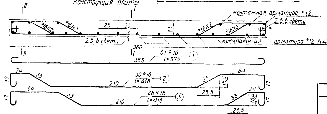
Конструкция плиты
