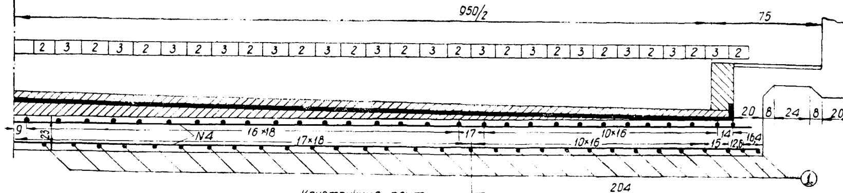
Конструкция плиты
