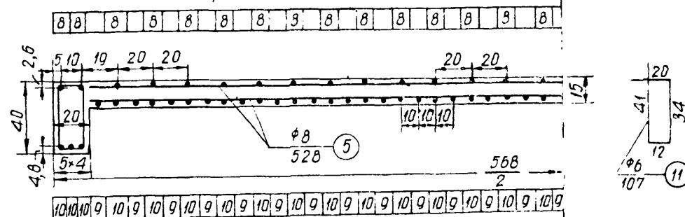
Продольный разрез III-III
