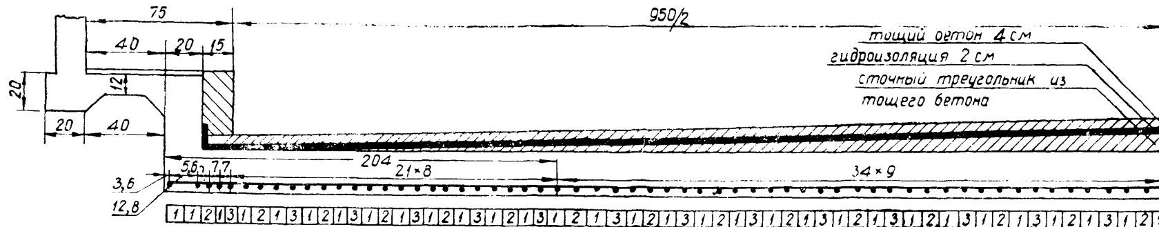
Разрез в пролете I-I
