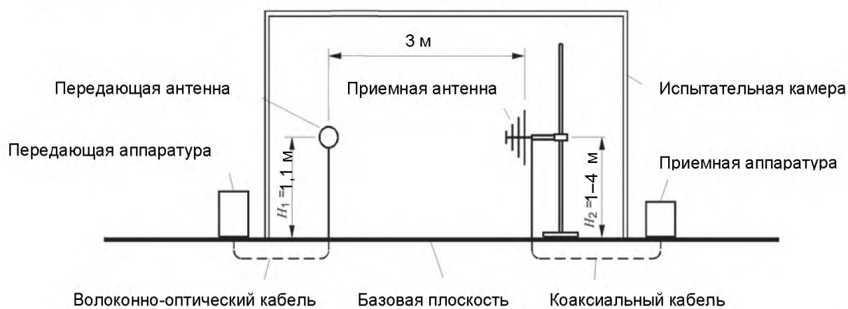
Рисунок 6 – Установка для измерения силы сигнала эталонного поля E_1
