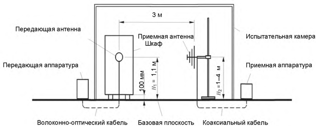
Рисунок 7 – Установка для измерения рассеяния силы сигнала поля E_2 (шкаф)
