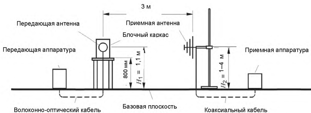
Рисунок 5 – Установка для измерения рассеяния силы сигнала поля E_2 (блочный каркас) 3.5.3 Полубезэховые или полностью безэховые камеры
