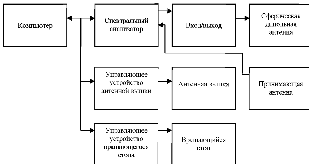
Рисунок 1 – Типовая установка для испытаний (как указано на рисунках с 3 по 8, антенны должны быть выбраны, как описано в 3.3.2 и 3.3.3)
