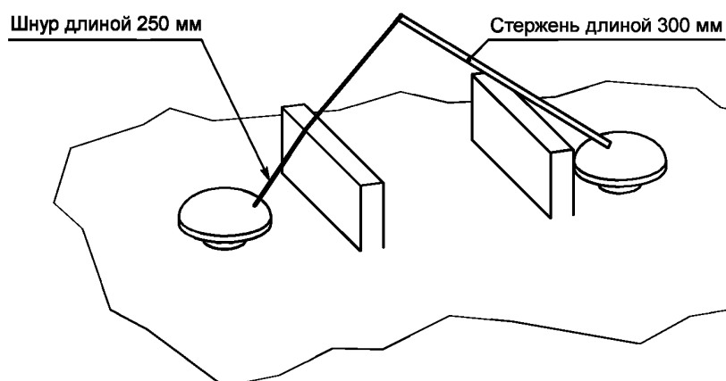
Рисунок А.5 — Разделение разделительными защитными устройствами
