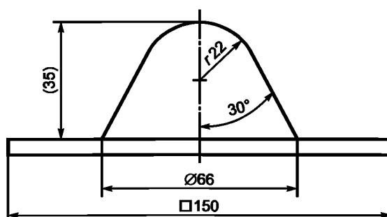
Рисунок А.7 — Размеры испытательного конуса
