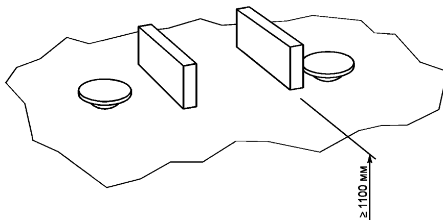
Рисунок А.11 — Предотвращение несанкционированного включения месторасположением
