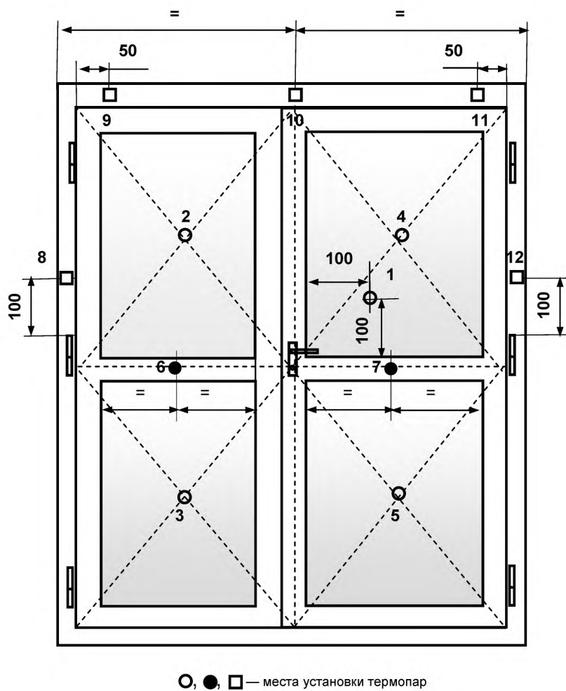
Рисунок А.7 — Схема установки термодатчиков на необогреваемой поверхности двухпольного дверного блока
