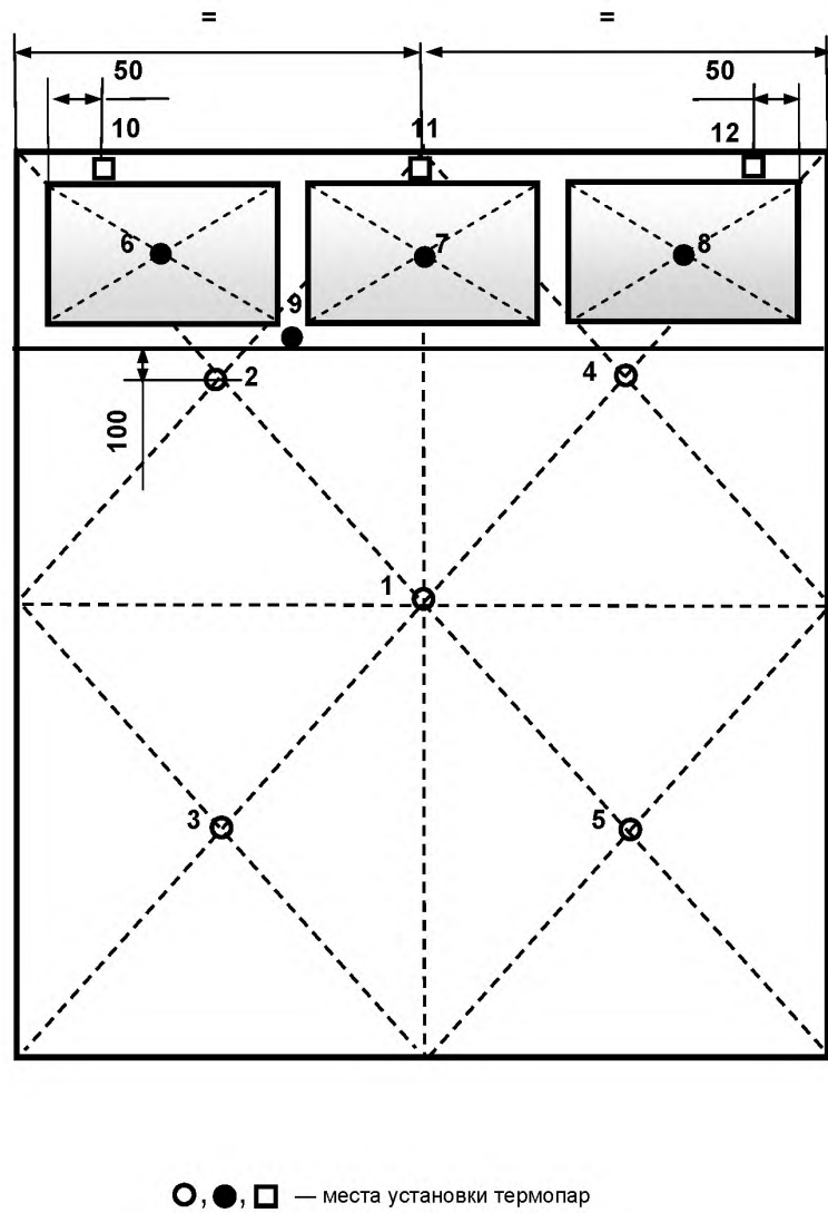
Рисунок А.4 — Схема установки термопар на необогреваемой поверхности перегородки
