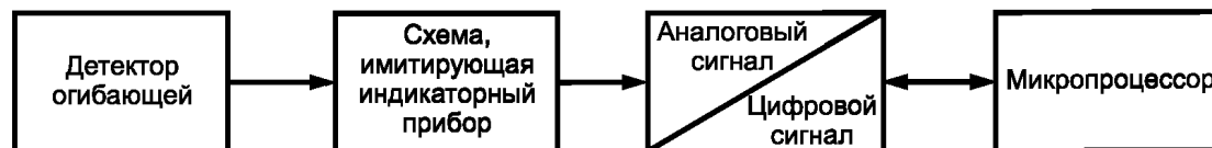
Рисунок 4 — Блок-схема детектора средних значений
