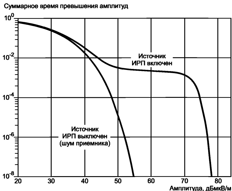
Рисунок G.3 — Пример функции распределения амплитуд ИРП
