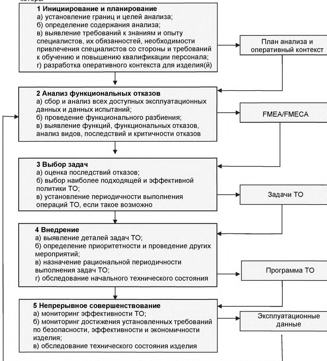
Рисунок 1 – Обзор процесса RCM
