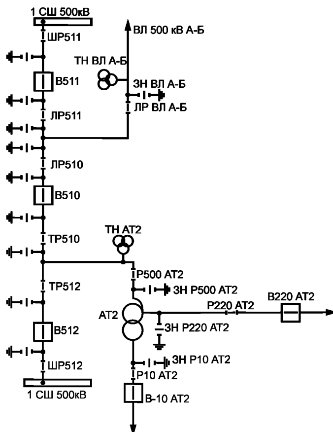
Рисунок Е.3 — Схема ПС 500 кВ, выполненная по полупортретной схеме
