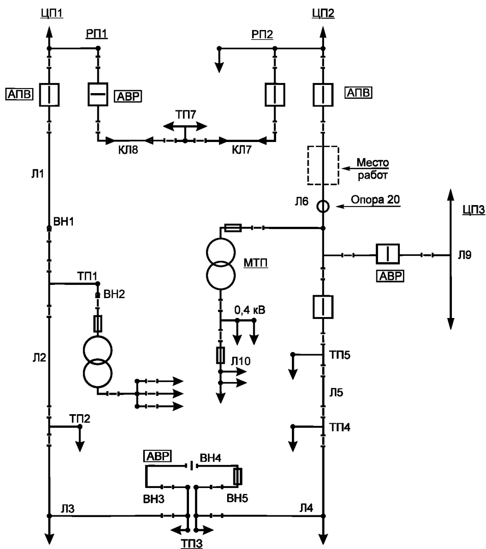
Рисунок Ж.2 — Схема участка распределительной электросети 6—10 кВ, секционированной в ТПЗ в нормальном режиме работы
