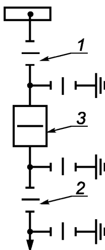
1 — шинный разъединитель; 2 — линейный разъединитель; 3 — выключатель
