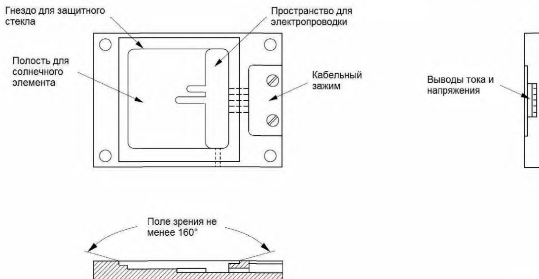
Рисунок 2 – Корпусирование одиночного солнечного элемента.
