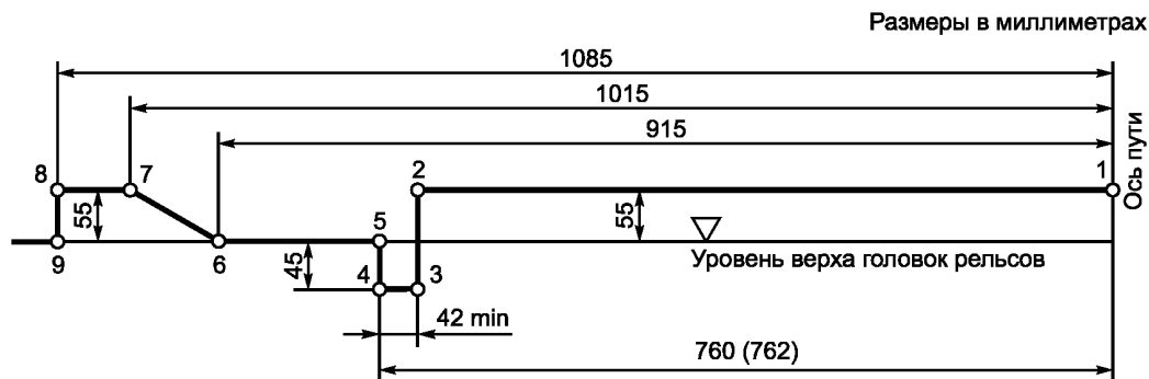
Рисунок 27 — Нижнее очертание габаритов C и C_n для двойных перекрестных стрелочных переводов, планок контроля нижнего габарита, устройств контроля схода подвижного состава
