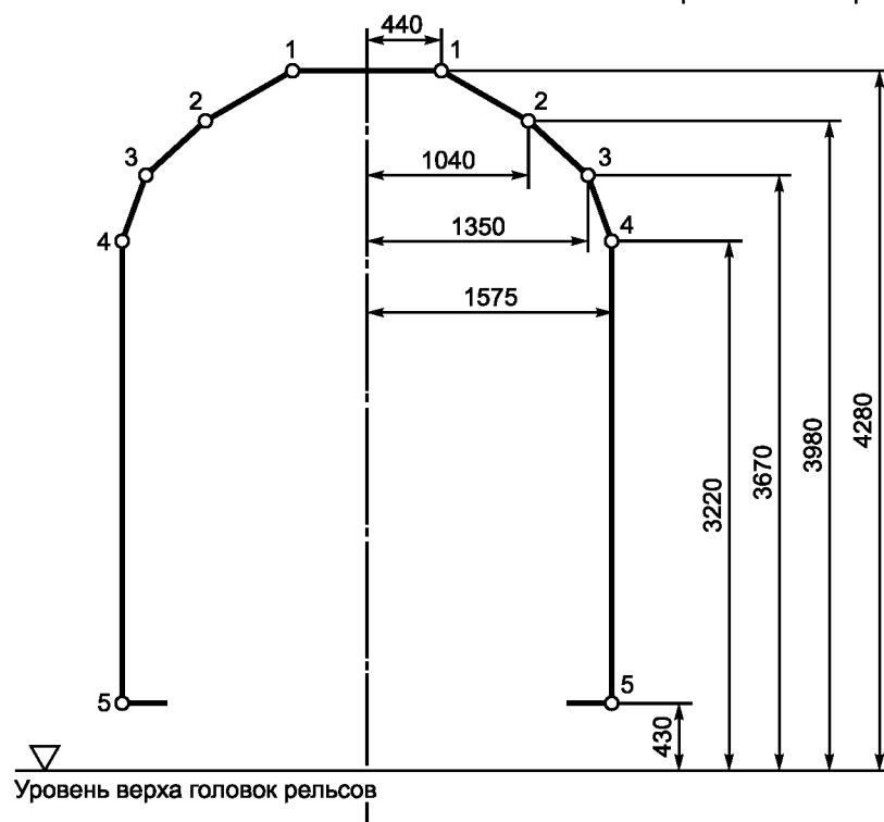
Рисунок 13 — Статический габарит 03- BM_{st}
