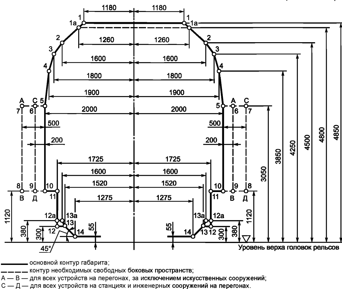
Рисунок Б.1 — Верхнее очертание габарита 1-СМ
