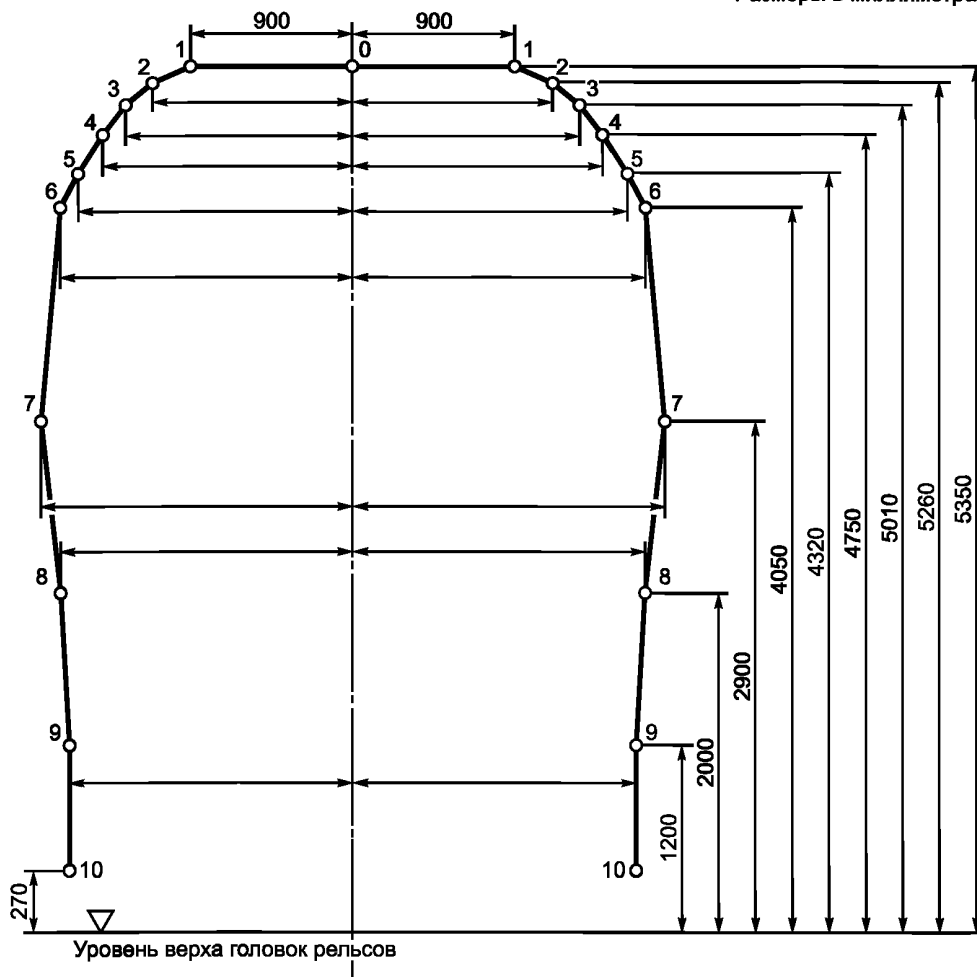
Рисунок Г.2 — Контрольное очертание сооружений Ц для пропуска подвижного состава габарита T_{\text{ц}} при скорости движения более 40 км/ч
