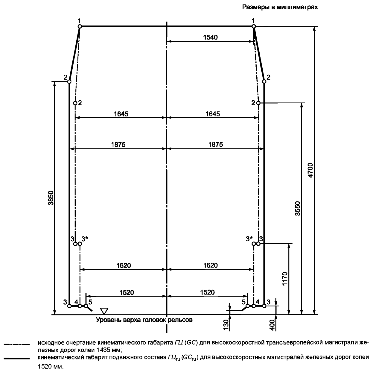
Рисунок 9 — Габарит подвижного состава \Gamma\zeta ( GC ) и гармонизированный с ним габарит \Gamma\zeta_{\text{гу}} ( GC_{\text{гу}} )
