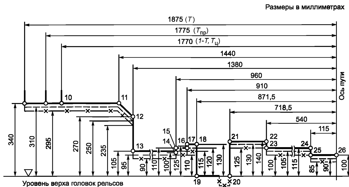
Рисунок 7 — Нижнее очертание габаритов для подвижного состава, проходящего по сортировочным горкам, оборудованным вагонными замедлителями при любом их положении
