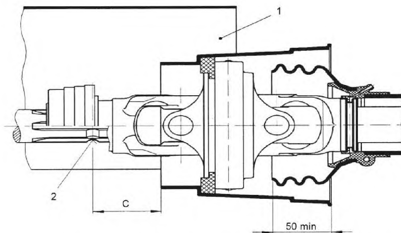
1 – защитный козырек BOM трактора; 2 – ось блокирующего устройства
