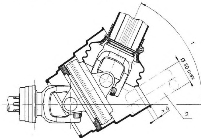
1 – максимальный угол складывания карданного вала; 2 – контрольный калибр диаметром Ø 31 мм
